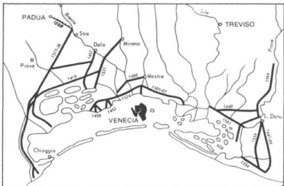
FIGURA 4. Los canales de regularización han salvaguardado la mitad de las lagunas venecianas.
