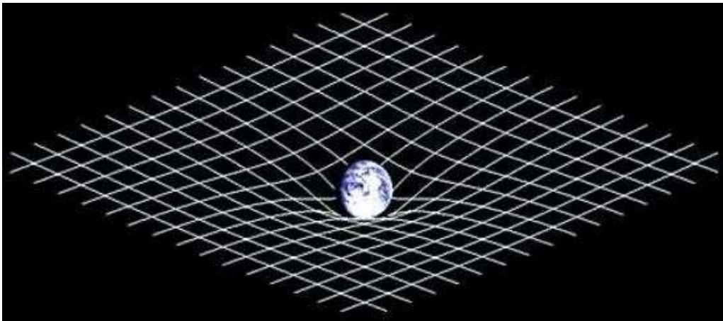
Representación esquemática de la distorsión de un espacio plano por un objeto de gran masa, que ayuda a entender la gravitación y los agujeros negros.
