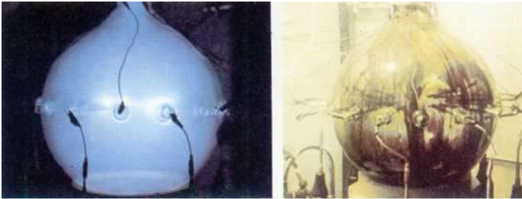
Síntesis de materia orgánica en el Laboratorio de Estudios Planetarios de la Universidad de Cornell. Primeras chispas eléctricas en una mezcla transparente de los gases metano, amoníaco, sulfuro de hidrógeno y agua en un frasco de cristal (izquierda). Al cabo de unas pocas horas de chispas, el interior del frasco queda recubierto (derecha) por una rica variedad de moléculas orgánicas de importancia para el origen de la vida. (Cedidas por Bishun Khare.)
