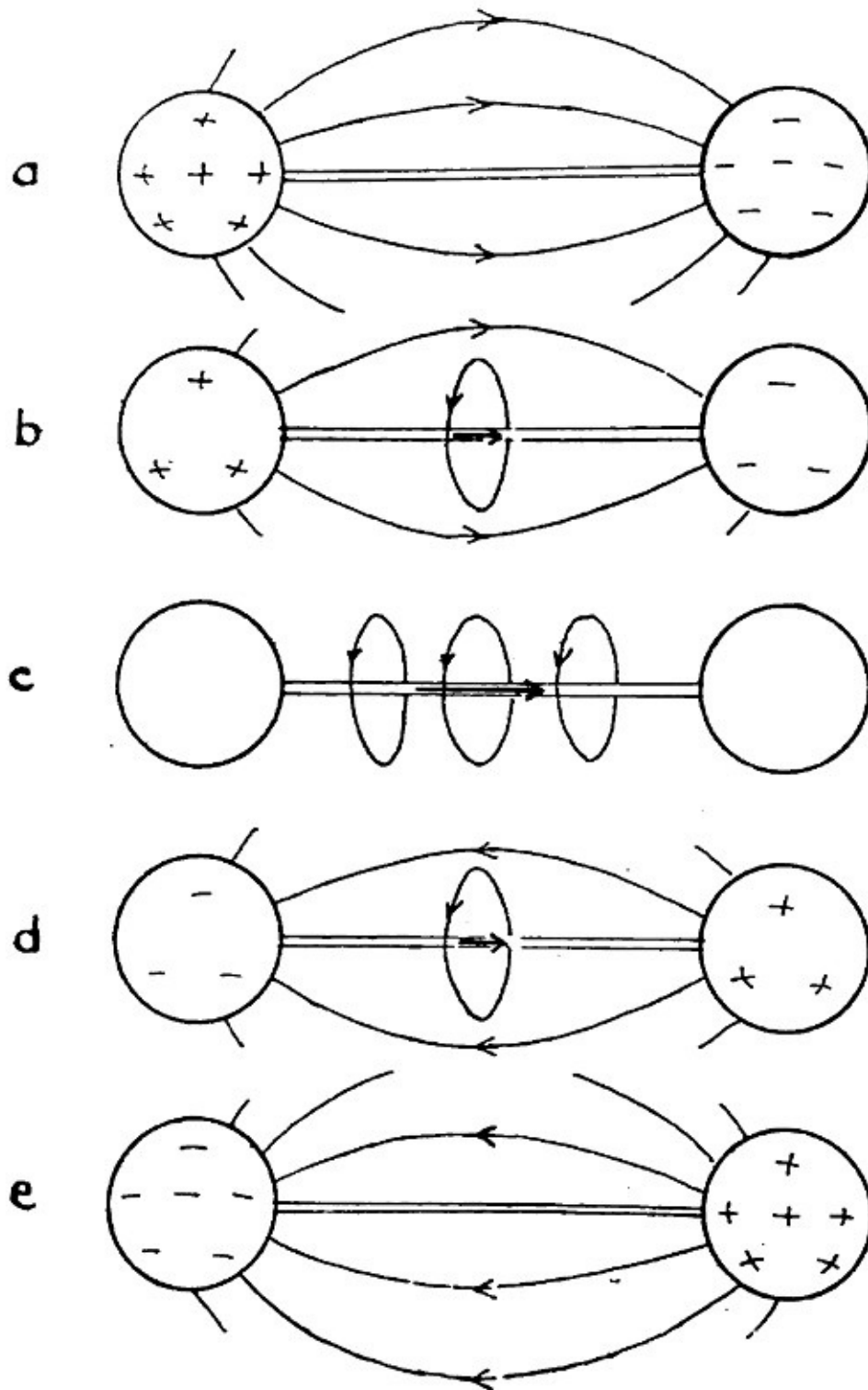
Figura 5.17. Oscilaciones electromagnéticas entre dos conductores en que la energía del campo eléctrico (a) se transforma periódicamente en la energía del campo magnético (c), y viceversa (e).
