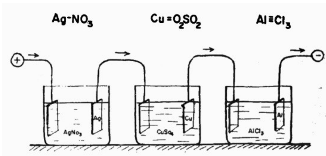
Figura 5.10. Demostración de las leyes de la electrólisis de Faraday. Si se hace pasar una corriente eléctrica a través de soluciones de nitrato de plata, sulfato de cobre y cloruro de aluminio, los metales se depositan en los electrodos negativos. La cantidad de metales depositados es proporcional a la cantidad de electricidad que pasa a través de las soluciones (primera ley de Faraday). También vio que si la cantidad de plata depositada es de 108 gramos (peso atómico de la plata), la cantidad de cobre depositado es sólo de 31,7 gramos (la mitad del peso atómico del cobre) y la cantidad de aluminio depositado es sólo de 9 gramos (un tercio del peso atómico del aluminio). Como la misma cantidad de electricidad pasa a través de los tres vasos, se deduce que el ion de cobre transporta el doble de la carga eléctrica transportada por el ion de plata, y el ion de aluminio transporta tres veces más. Esto coincide con la equivalencia química de los tres metales, como se ve en las fórmulas que figuran en la parte superior del diagrama. Esta es la segunda ley de Faraday.
