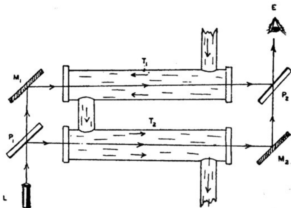
Figura 6.2. Experimento de Fizeau para observar el cambio de la velocidad de la luz cuando se propaga en un medio en movimiento.
