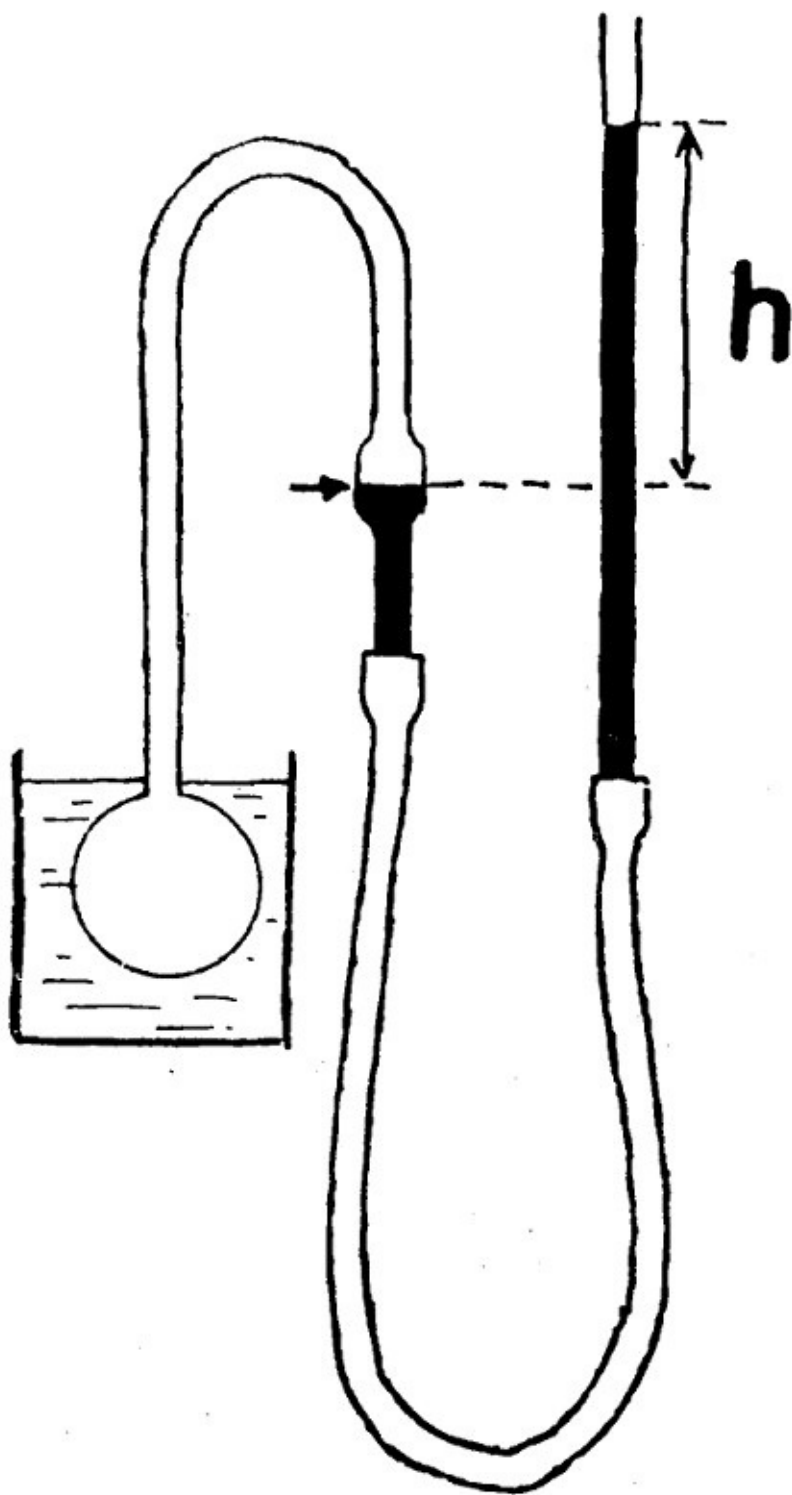
Figura 4.2. Principio del termómetro de gas. Cuanto más alta es la temperatura del líquido en la vasija de la izquierda, más alto es el nivel h del mercurio en el tubo móvil de la derecha, de suerte que el nivel del mercurio en el tubo del centro queda en el mismo lugar indicado por la flecha.
