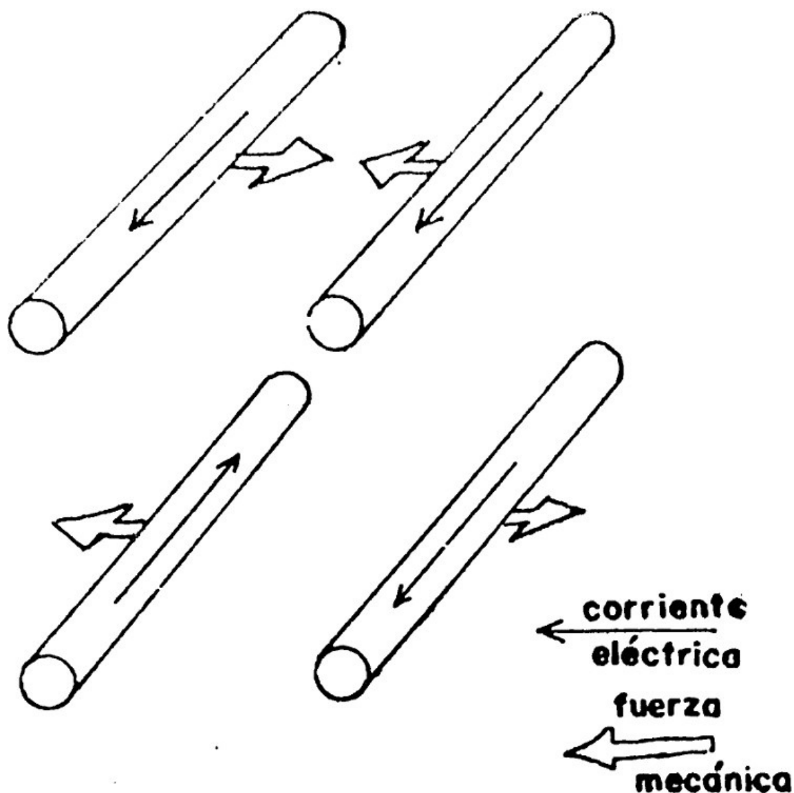
Figura 5.7. Leyes de Ampère de la interacción entre corrientes.
