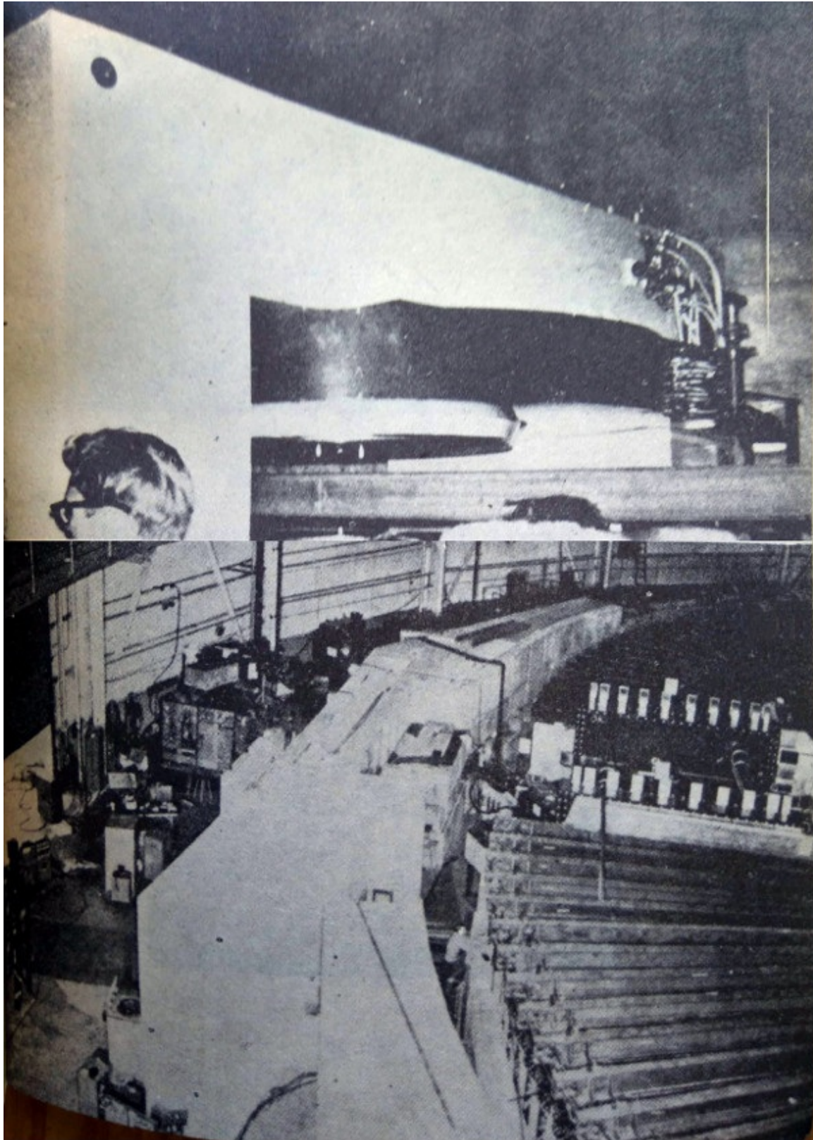
Lámina VI. (Arriba.) Ciclotrón de la Universidad de Colorado en el que se ve un polo del electroimán y el haz de partículas. (Abajo.) Una sección del bevatrón de la Universidad de California.
