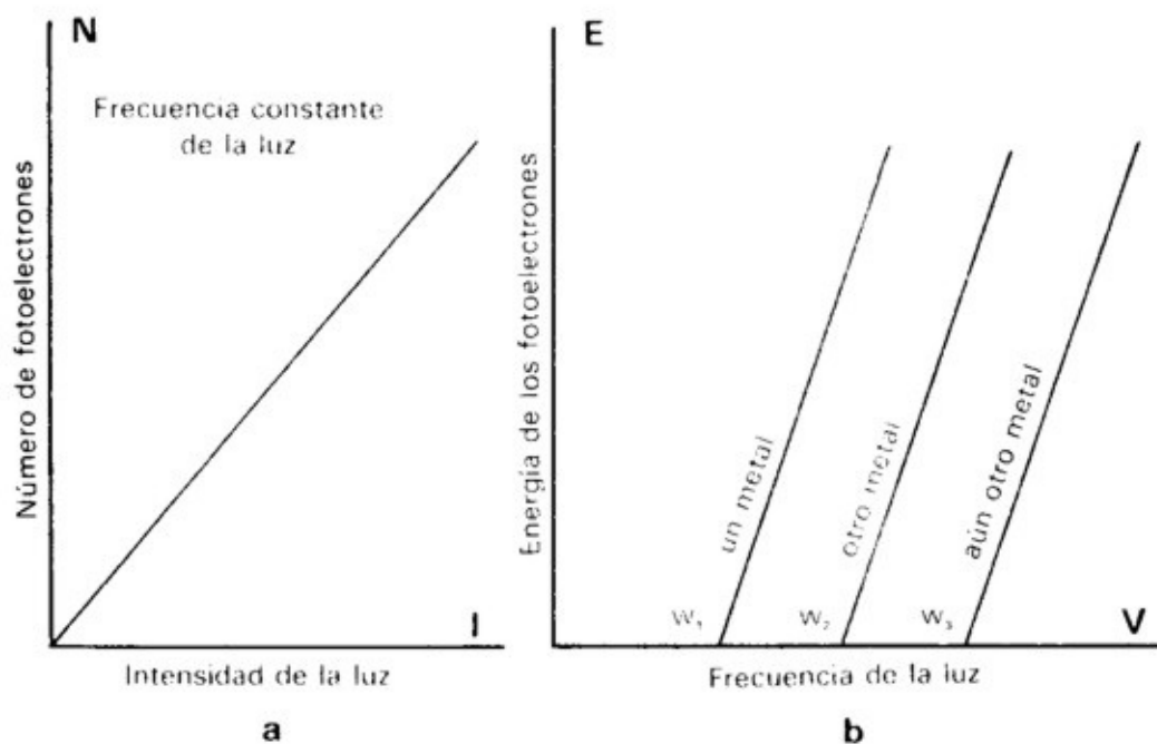
Figura 7.11. Leyes del efecto fotoeléctrico halladas experimentalmente. a) La dependencia entre el número de fotoelectrones y la intensidad de la luz. b) La dependencia entre la energía de los
