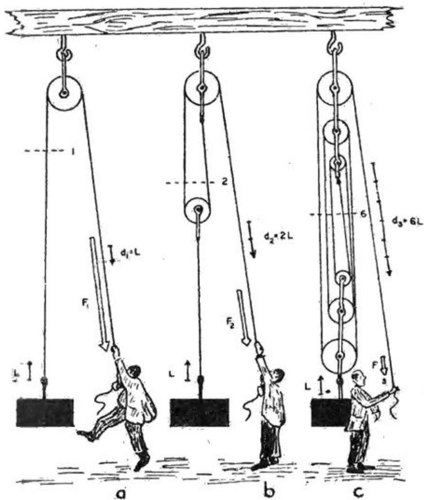
Figura 1.5. El principio de la polea.
