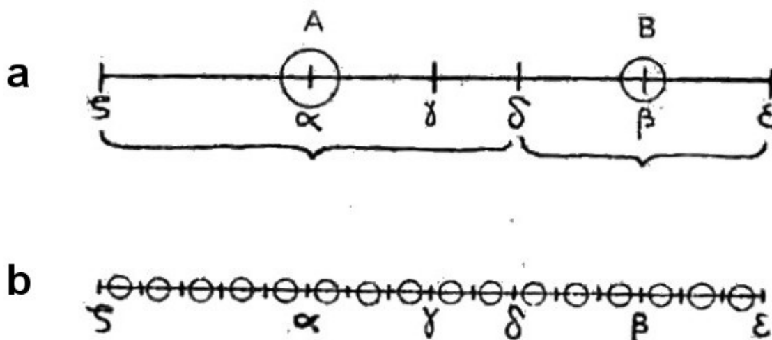
Figura 1.3. Prueba arquimédica de la ley de la palanca.
