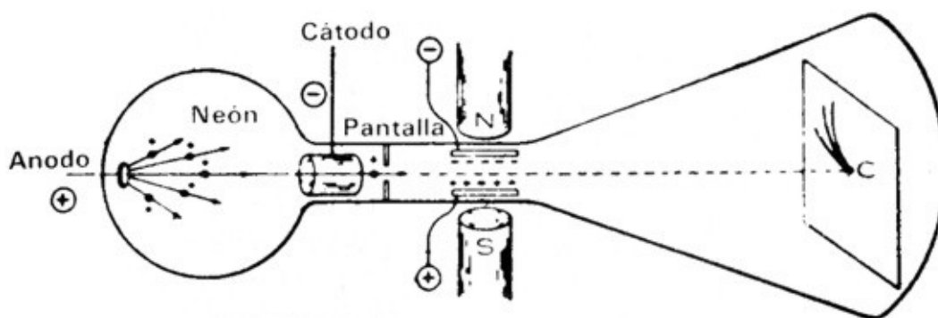
Figura 7.5. Aparato de Thomson para el estudio de los rayos canales. Los iones positivos que se mueven del ánodo al cátodo pasan a través de canales abiertos en el cátodo, y después de pasar por una pantalla entran en la región del campo eléctrico y magnético orientados en la misma dirección. Como la desviación magnética (en la dirección horizontal) depende de la velocidad de las partículas, mientras que la desviación eléctrica (en dirección vertical) depende del cuadrado de esta velocidad, las partículas de la misma masa, pero que se mueven con velocidades diferentes, serán distribuidas a lo largo de una parábola en la pantalla C.
