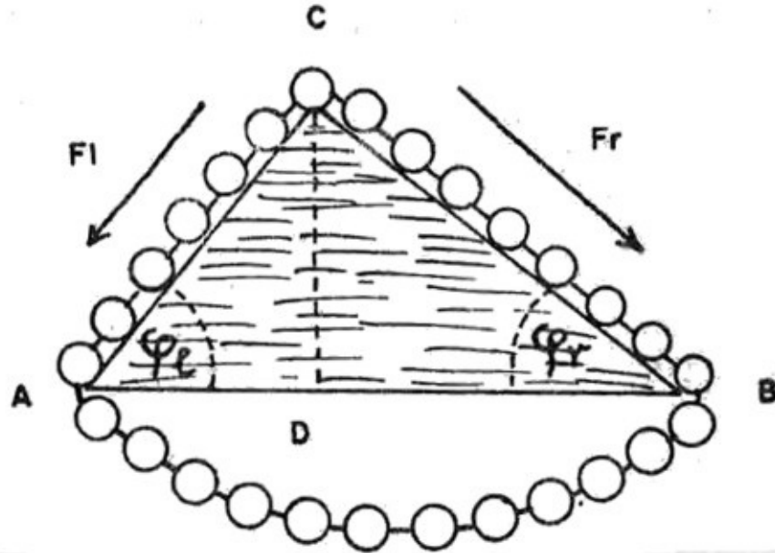
Figura 2.3. La cadena sin fin de Stevinus demostrando la ley de equilibrio en un plano inclinado.
