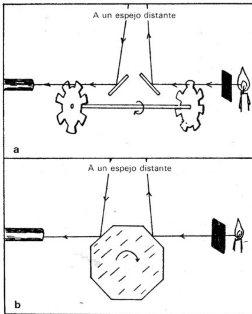
Figura 6.1. Métodos de Fizeau (a) y Foucault (b) para la medida de la velocidad de la luz.
