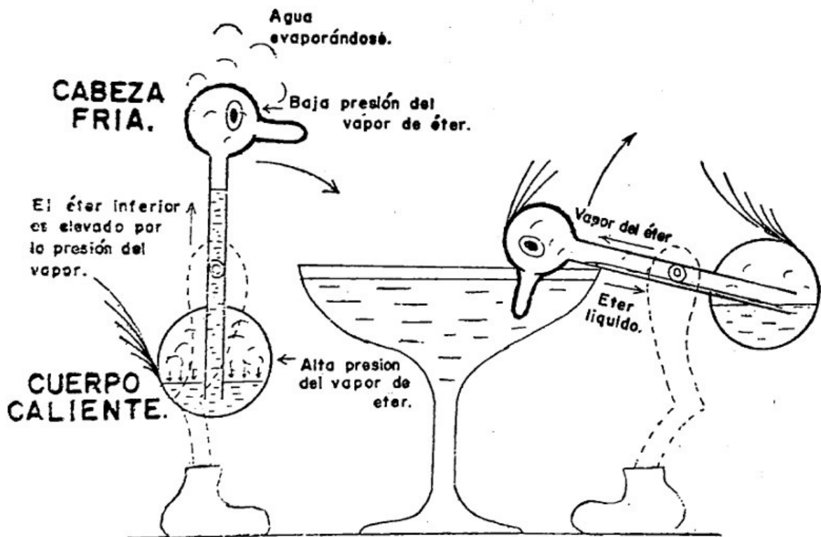
Figura 4.7. Los pájaros bebedores japoneses.
