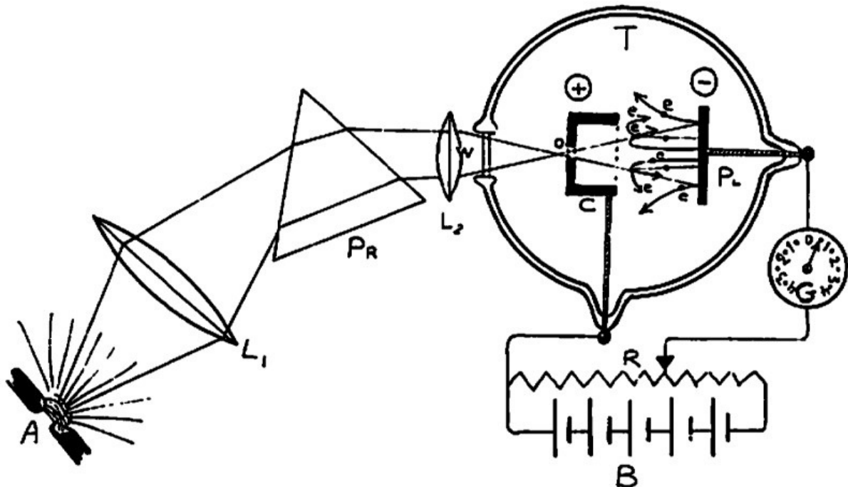
Figura 7.10. Aparato para el estudio del efecto fotoeléctrico. Los fotoelectrones proyectados por la lámina P_L hacia el cilindro C son detenidos por el campo eléctrico si la diferencia de potencial entre P_L y C es bastante grande.
