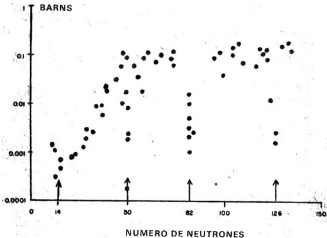
Figura 8.13. «Sección eficaz de captura» de neutrones como función del número de neutrones en el núcleo.
