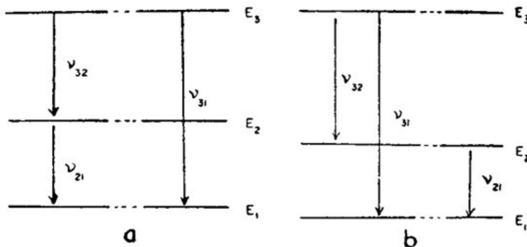
Figura 7.12. Ilustración del principio de Rydberg. a) Si un electrón puede saltar del nivel de energía E_3 al nivel E_2 emitiendo la frecuencia \nu_{32} y saltar otra vez de E_2 a E_1 emitiendo la frecuencia \nu_{21} , entonces debe ser también posible una transición directa de E_3 a E_1 emitiendo la frecuencia \nu_{31} = \nu_{32} + \nu_{21} . b) Si un electrón salta de E_3 a E_2 emitiendo la frecuencia \nu_{32} o a E_1 emitiendo la frecuencia \nu_{31} , también debe ser posible la transición de E_2 a E_1 con la frecuencia \nu_{21} = \nu_{31} - \nu_{32} .
