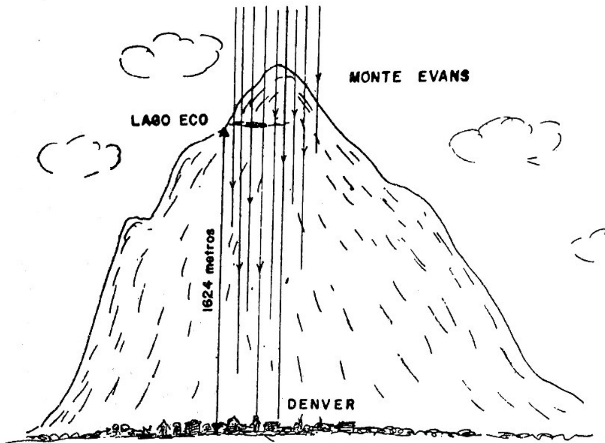
Figura 8.20. Desintegración de los mesones en su descenso desde el Lago Eco a Denver.
