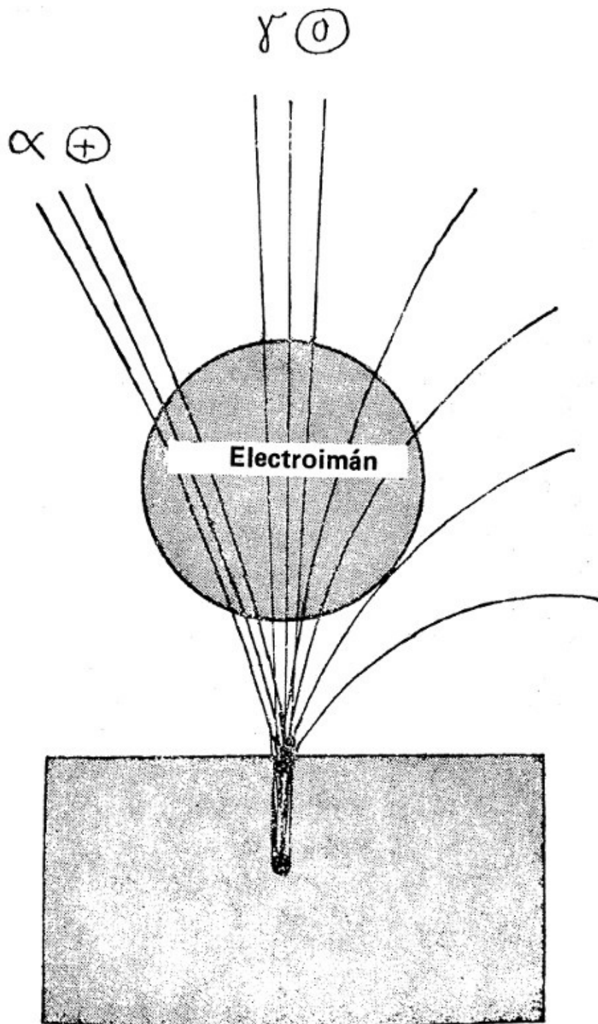
Figura 8.1. Rayos alfa, beta y gamma
