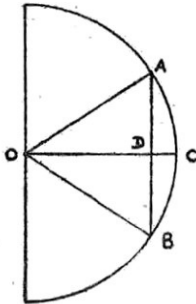
Figura 1.11. La relación entre las tablas de las cuerdas de Plutarco y las modernas tablas trigonométricas. Plutarco establecía las longitudes de las cuerdas ADB para las diversas longitudes de los arcos ACB. En la trigonometría moderna se tabula la longitud AD (media cuerda) en función del arco AC. La longitud AD se llama seno y la longitud OD coseno del ángulo AOC.
