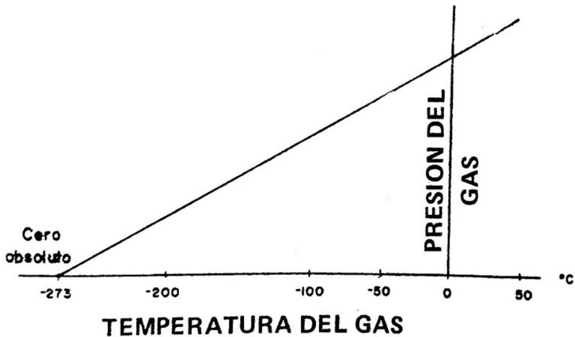
Figura 4.3. Un gráfico que muestra la dependencia de la presión de un gas (contenido en un volumen dado) de la temperatura. A la de -273 grados la presión del gas es cero.
