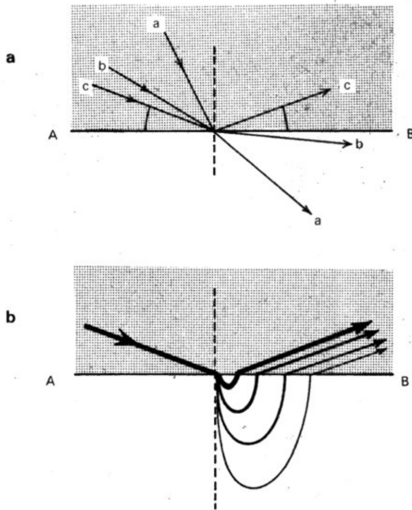
Figura 8.4. Reflexión total interna de la luz, según la óptica geométrica (a) y según la óptica ondulatoria (b).
