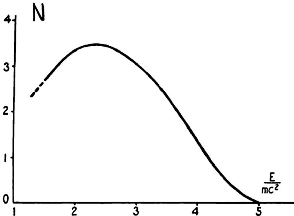
Figura 8.7. El espectro de rayos \beta del \text{In}^{114} . El número ( N ) de electrones aparece en función de la energía ( E ) expresada en unidades de mc^2 .
