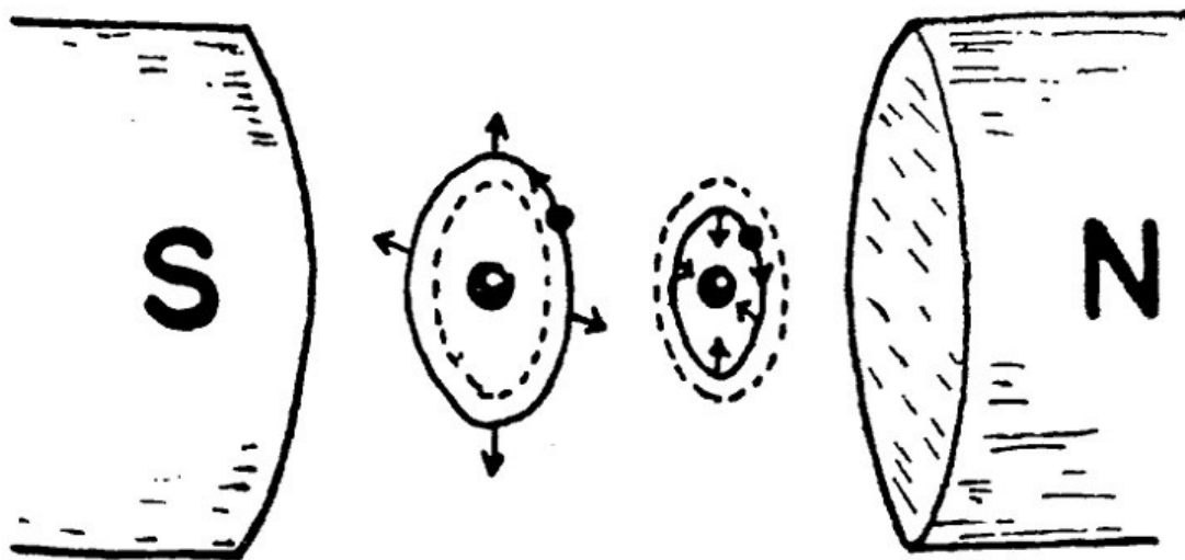
Figura 5.14. Explicación del «efecto Faraday». La fuerza que actúa sobre un electrón atómico que se mueve en un campo magnético depende de la dirección de su movimiento. En el caso de una rotación en sentido contrario a las agujas del reloj (izquierda), la fuerza aumenta el radio de la órbita y disminuye la frecuencia. En el caso de una rotación en el mismo sentido que las agujas del reloj (derecha), la fuerza disminuye el radio e incrementa la frecuencia. Interactuando con la luz, estos dos tipos de movimiento electrónico hacen girar el plano de polarización.
