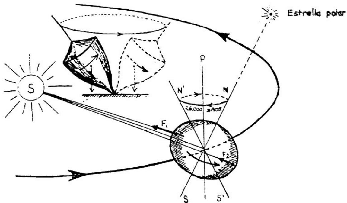
Figura 3.4. Explicación de Newton de la precesión del eje de rotación de la Tierra. Como la fuerza de la gravedad disminuye con la distancia, la fuerza F_1 , actuando sobre el abultamiento ecuatorial que mira hacia el Sol, es mayor que la fuerza F_2 , que actúa en el lado opuesto más lejano. Así, la acción combinada de las dos atracciones ejerce una «fuerza enderezadora» sobre el eje de rotación, es decir, tiende a colocarlo perpendicular al plano de la órbita. La situación es similar a la que existe en el caso de un trompo giratorio con un eje inclinado, en el que la fuerza de la gravedad, es decir, su peso, tiende a hacer horizontal su eje. Y del mismo modo que el trompo no se cae mientras está girando, sino que queda erguido con su eje describiendo una superficie cónica en torno a la vertical, el eje de la Tierra no se sitúa perpendicularmente a la órbita, sino que describe una superficie cónica en torno a esa dirección.
