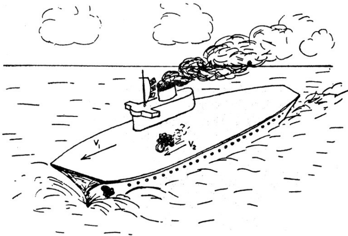
Figura 6.8. Suma relativista de dos velocidades.
