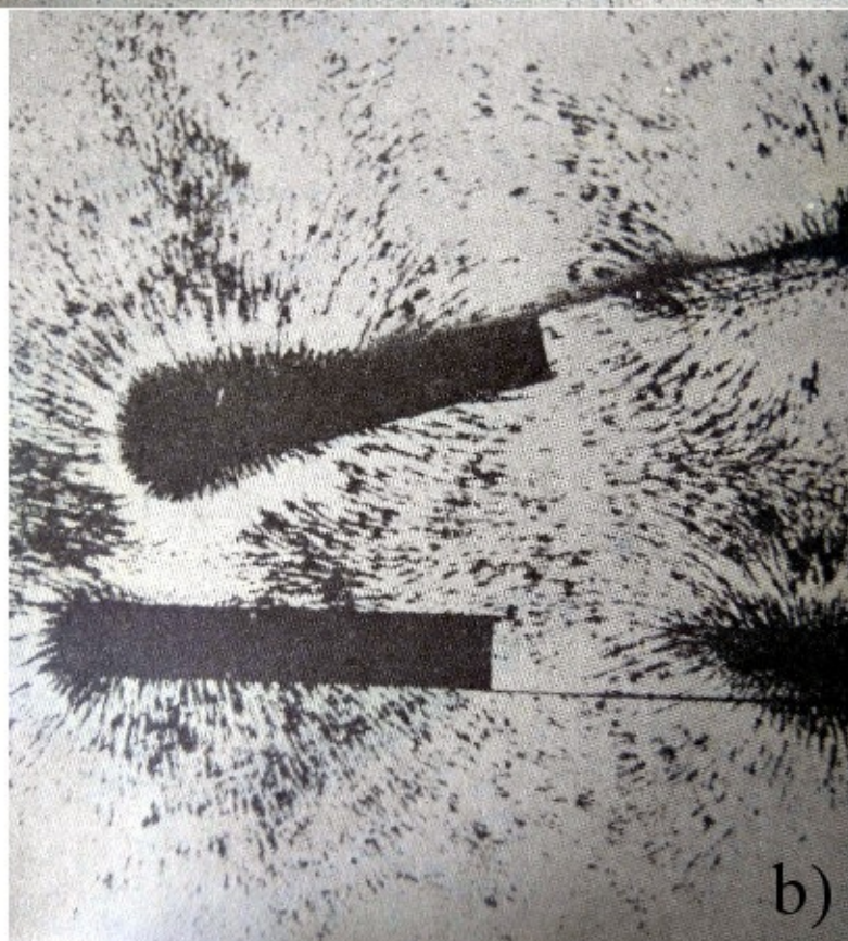
Lámina III. a) Líneas magnéticas de fuerza entre dos imanes orientados en direcciones opuestas. b) Líneas magnéticas de fuerza entre dos imanes orientados en la misma dirección.
