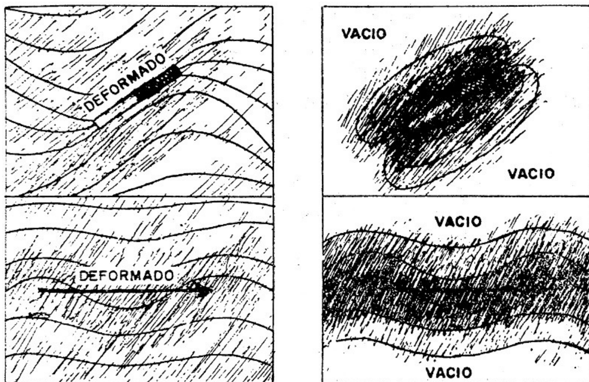
Figura 6.9. El viejo y el nuevo concepto de campo electromagnético. Antes de Einstein se creía que el éter que penetra todo el mundo se deformaba en la región del campo electromagnético. Ahora creemos que el campo electromagnético es una entidad física (ponderable) que existe por sí misma en un espacio vacío.
