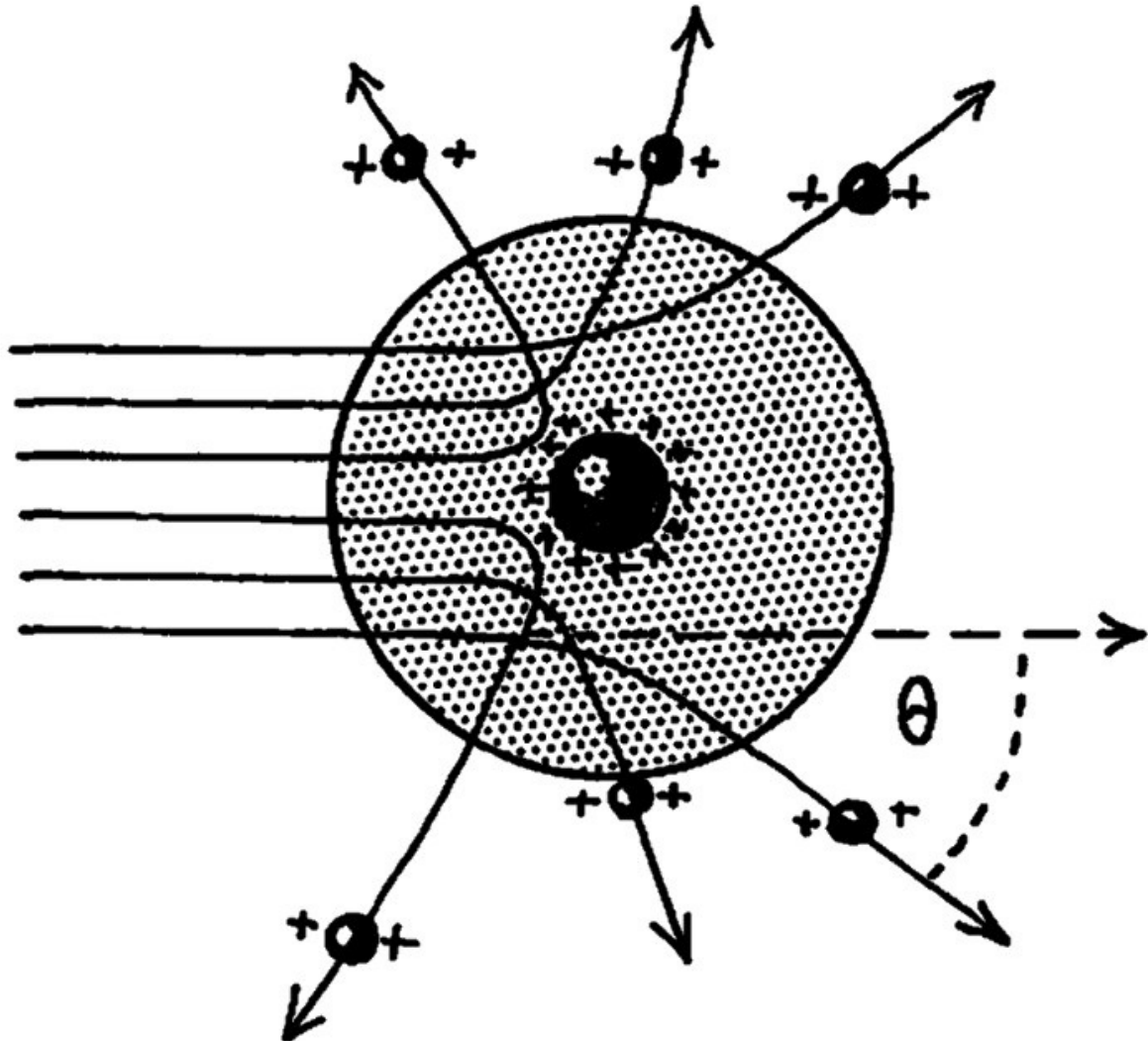
Figura 7.7. Modelo nuclear de un átomo.
