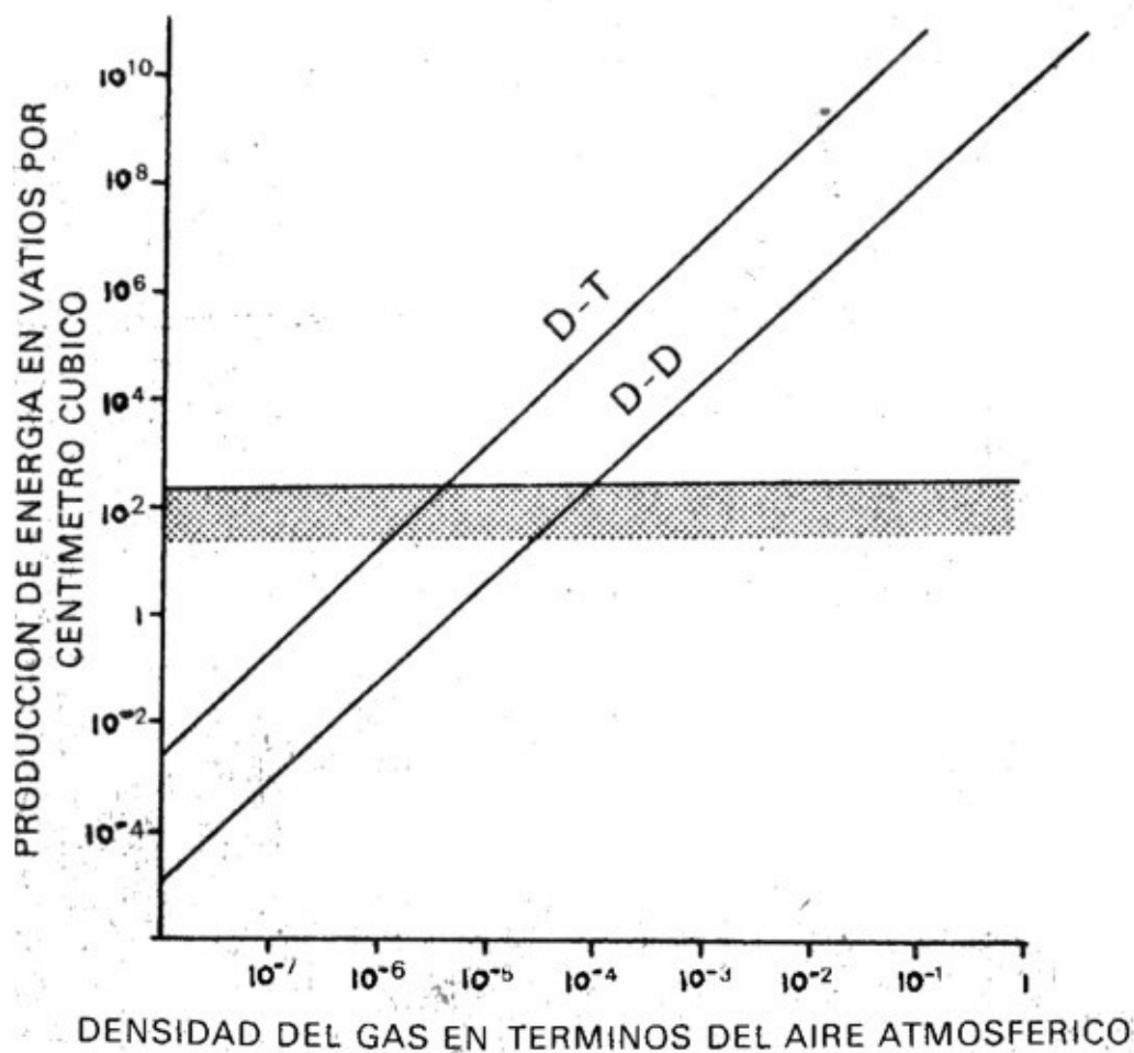
Figura 8.17. La tasa de liberación de energía nuclear para densidades variables del gas a la temperatura de 7 \times 10^9 K (unas dos veces la temperatura interior del Sol). La faja sombreada representa la producción de energía en los reactores de uranio y plutonio existentes.
