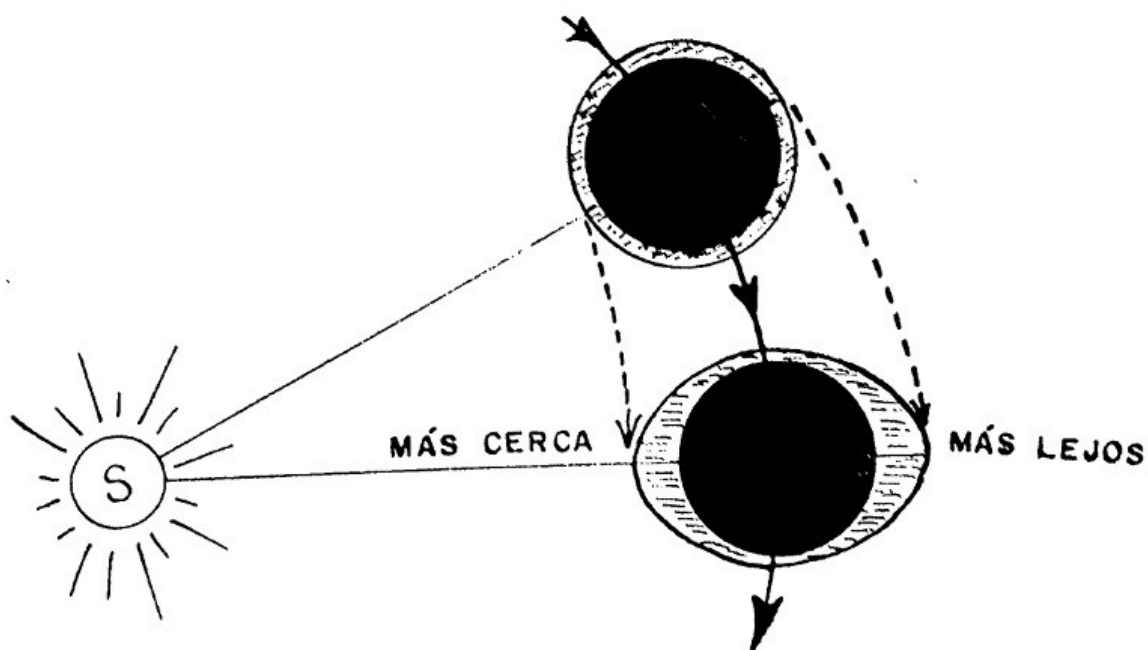
Figura 3.5. Explicación por Newton de las mareas oceánicas. Como la fuerza de la gravedad disminuye con la distancia al Sol, la fuerza que actúa sobre el agua del océano en el lado alumbrado de la Tierra es algo mayor que la que actúa sobre el cuerpo sólido. De modo parejo, la fuerza de la gravedad que actúa sobre el lado nocturno es algo menor que si actuase sobre el cuerpo sólido. Como resultado de estas diferencias, la superficie del agua en el lado iluminado tiene tendencia a elevarse sobre el fondo del océano, mientras que en el lado nocturno el fondo del océano es, por así decir, «succionado desde debajo» de la superficie del océano. Ambos efectos dan lugar a la formación de dos abultamientos del agua, que, en conjunción con la rotación de la Tierra en torno a su eje, se manifiestan como dos mareas que corren en torno a la Tierra en un periodo de veinticuatro horas.
