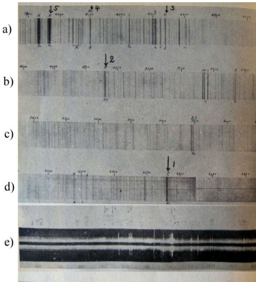
Lámina II. a), b), c), d). La parte visible del espectro solar tomado por un helioespectrógrafo de 13 pies. Las líneas numeradas corresponden al espectro de Balmer del hidrógeno. e) Espectro ultravioleta del Sol tomado desde un cohete volando a gran altura. Las líneas numeradas corresponden al espectro de Lyman del hidrógeno.
