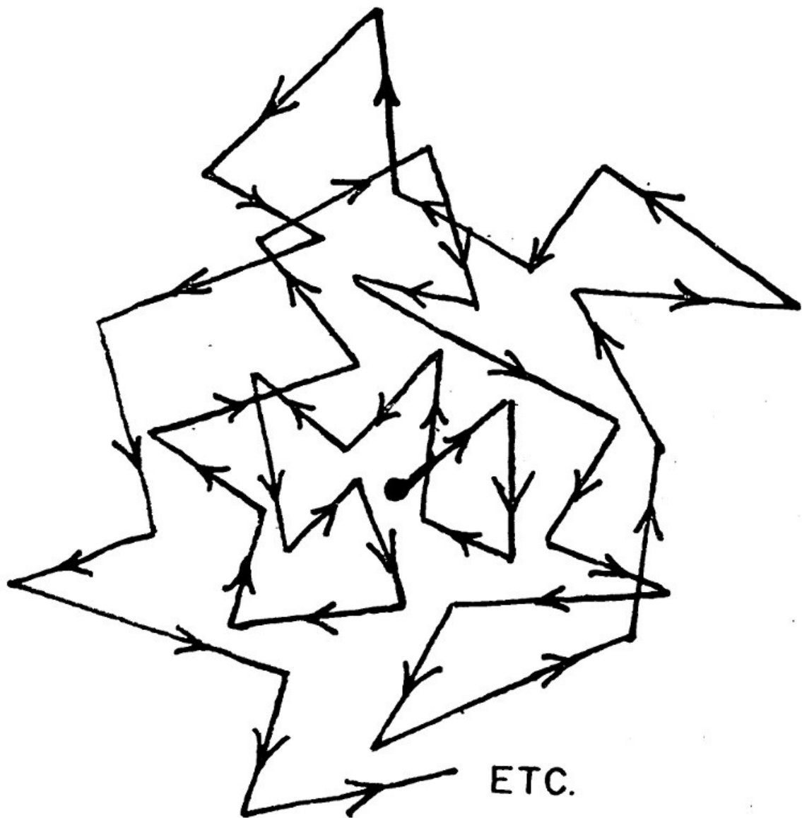
Figura 4.11. Una «trayectoria aleatoria» es el movimiento de un cuerpo cuya dirección cambia irregularmente como resultado del choque con otros cuerpos, ya sea una molécula que choca con otras o un borracho que choca con los faroles. Es evidente que, en este caso, el cuerpo avanza menos que si se moviera en línea recta, y puede demostrarse que la distancia media desde el punto inicial es igual a la longitud de cada paso en línea recta multiplicada por la raíz cuadrada del número de pasos.
