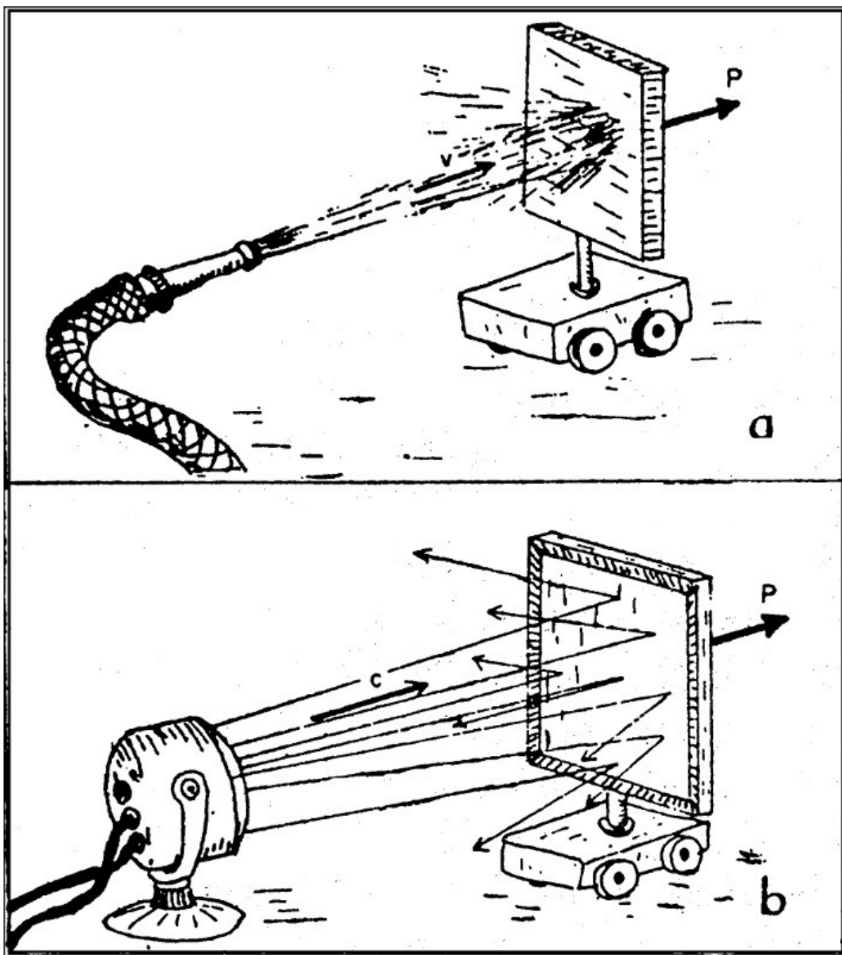
Figura 6.10. a) Reflexión de una corriente de agua por un tablero móvil, y b) la reflexión de un haz de luz por un espejo móvil.
