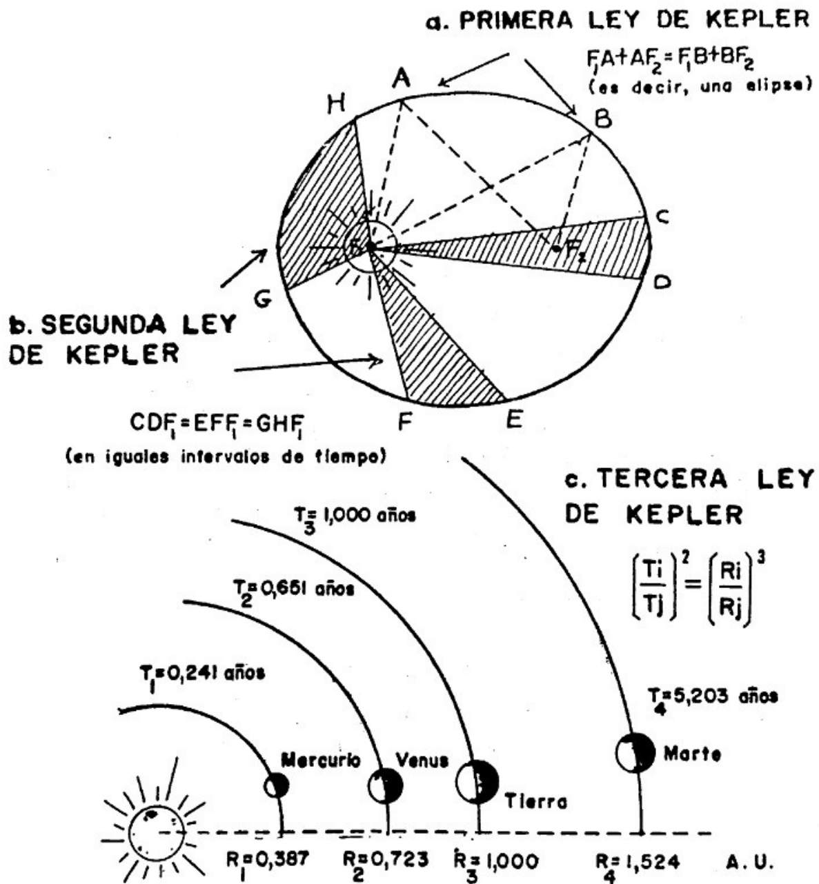
Figura 2.2. Las tres leyes de Kepler sobre el movimiento planetario.
