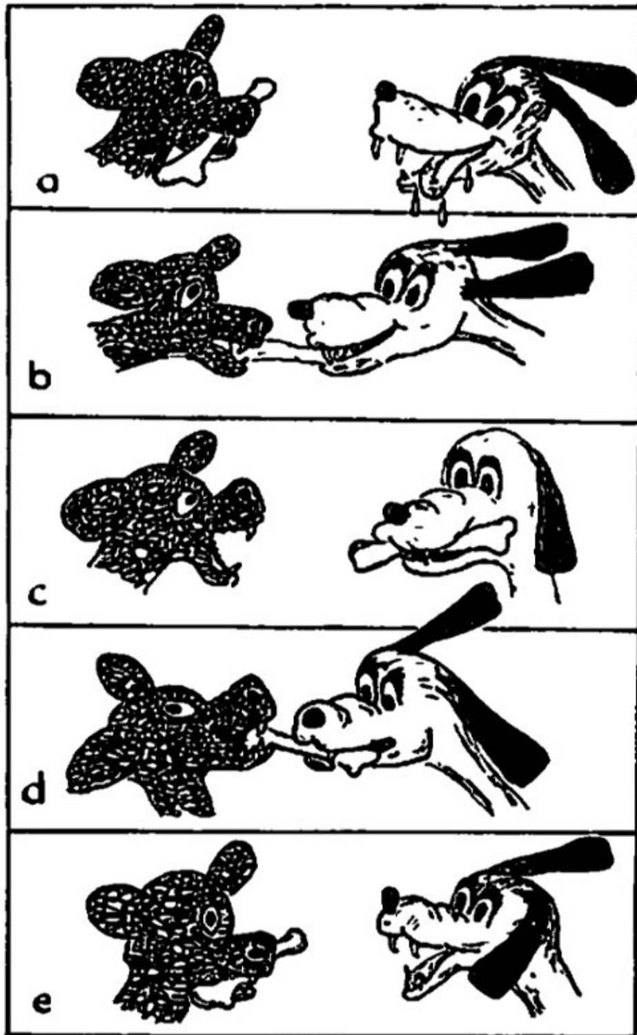
Figura 8.19. El intercambio de un mesón (el hueso) entre dos nucleones.
