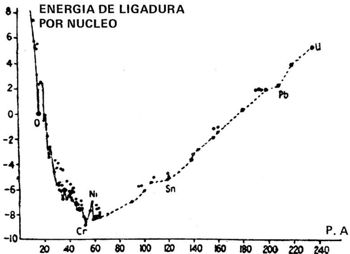
Figura 8.12. Energía de ligadura por nucleón como función del peso atómico.
