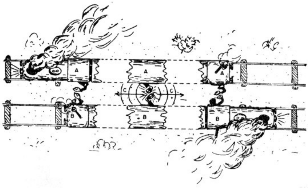
Figura 6.7. Sincronización de relojes en dos trenes que se mueven uno respecto al otro.
