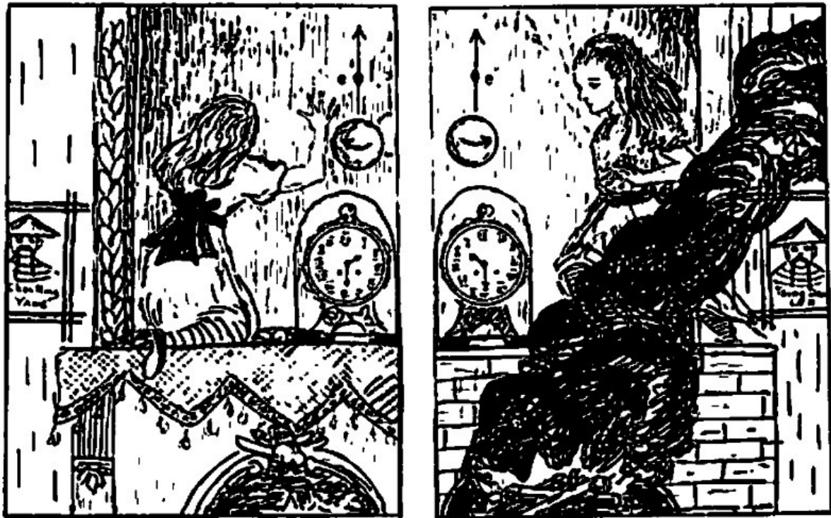
Figura 8.21. Imagen especular de la desintegración de un neutrón.
