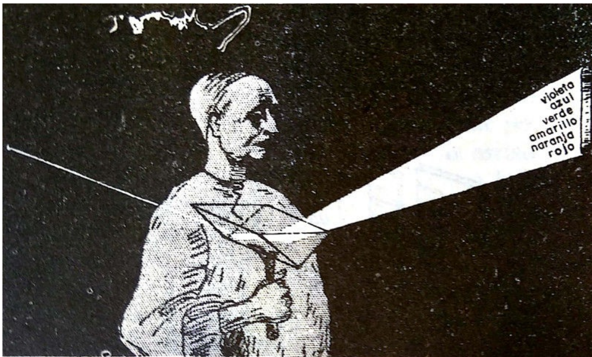
Figura 3.10. Sir Isaac Newton demuestra la descomposición de la luz en varios colores espectrales.
