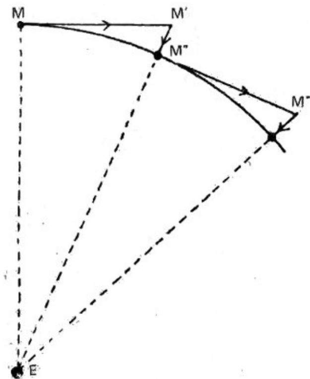
Figura 3.3. Considerando el movimiento circular de la Luna en torno de la Tierra como una caída continua (véase Figura 3.2), Newton pudo calcular la aceleración producida por la fuerza de la gravedad actuando sobre la Luna. El diagrama muestra cómo.
