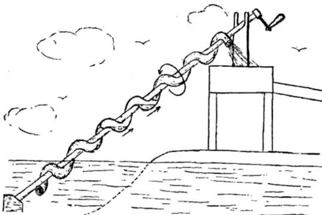
Figura 1.7. El tornillo de Arquímedes para elevar agua simplemente con hacerlo girar. Para comprender cómo funciona, piénsese lo que ocurre en las partes bajas del tubo cuando gira y se verá que ascienden, no el tubo mismo, sino las posiciones del contenido «mínimo» de agua. Puede ayudar a la comprensión hacer una espiral con un alambre metálico y ver lo que ocurre cuando gira alrededor de su eje.
