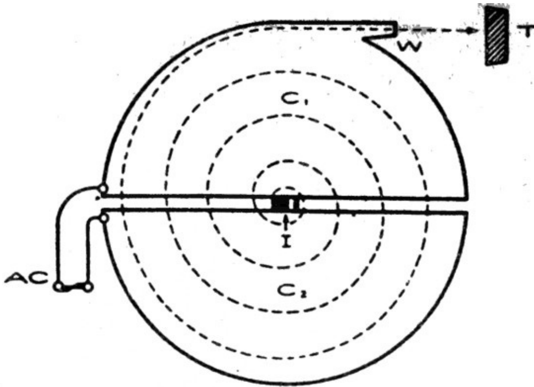
Figura 8.9. El principio del ciclotrón.
