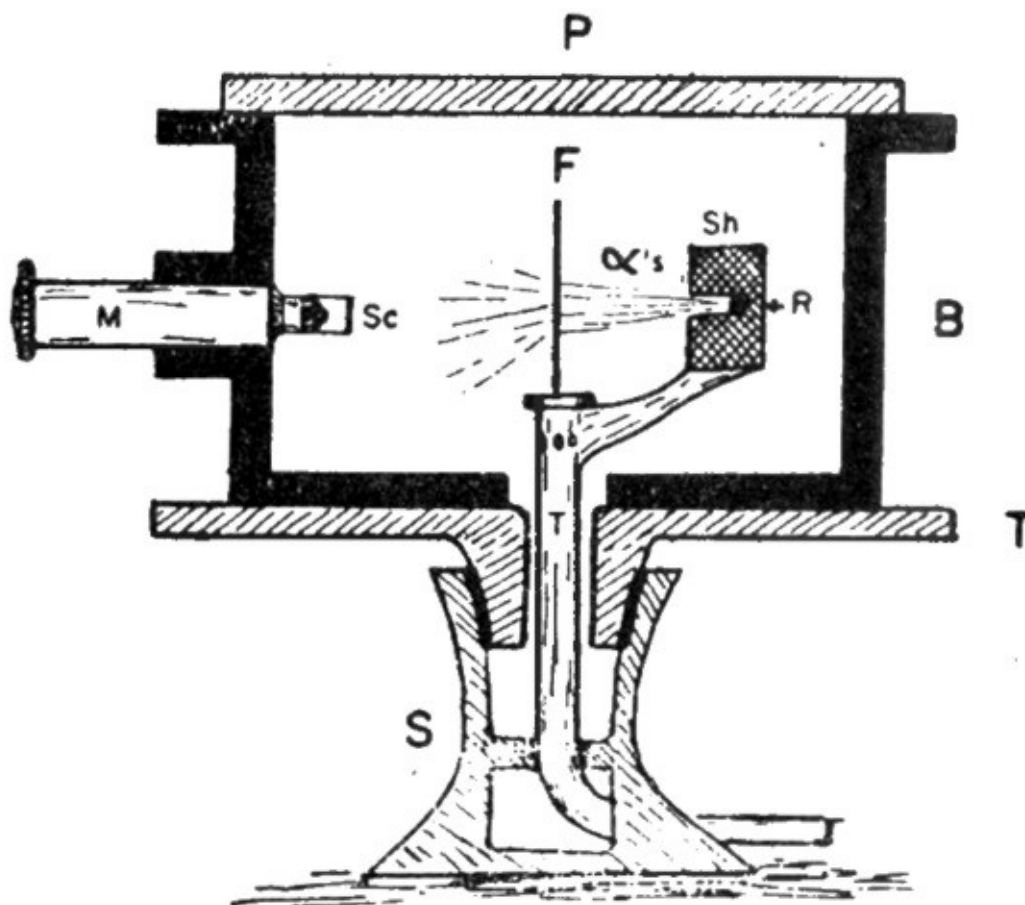
Figura 7.6. El primer aparato para el estudio de la dispersión de los rayos alfa. Una caja en que se ha hecho el vacío B, con una placa superior P movable está colocada sobre una mesa rotatoria T. La fuente radiactiva R, colocada en una lámina de plomo Sh, y el filamento F de dispersión están fijos al pedestal S. Un microscopio con la pantalla de centelleo Sc está fijo en la caja y puede girar en torno al eje horizontal.
