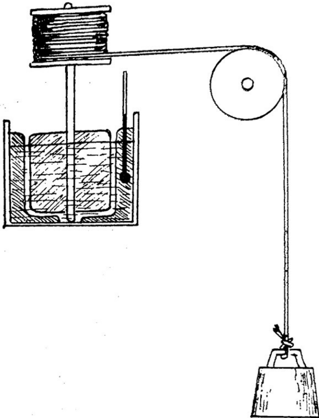
Figura 4.5. Experimento de Joule sobre la transformación de la energía mecánica en calor. El peso que descende hace girar las paletas en una vasija llena de agua y la temperatura del agua aumenta por el rozamiento interno. Comparando el trabajo realizado por el peso que descende con el aumento de calor del agua, Joule obtuvo el valor del equivalente mecánico del calor.
