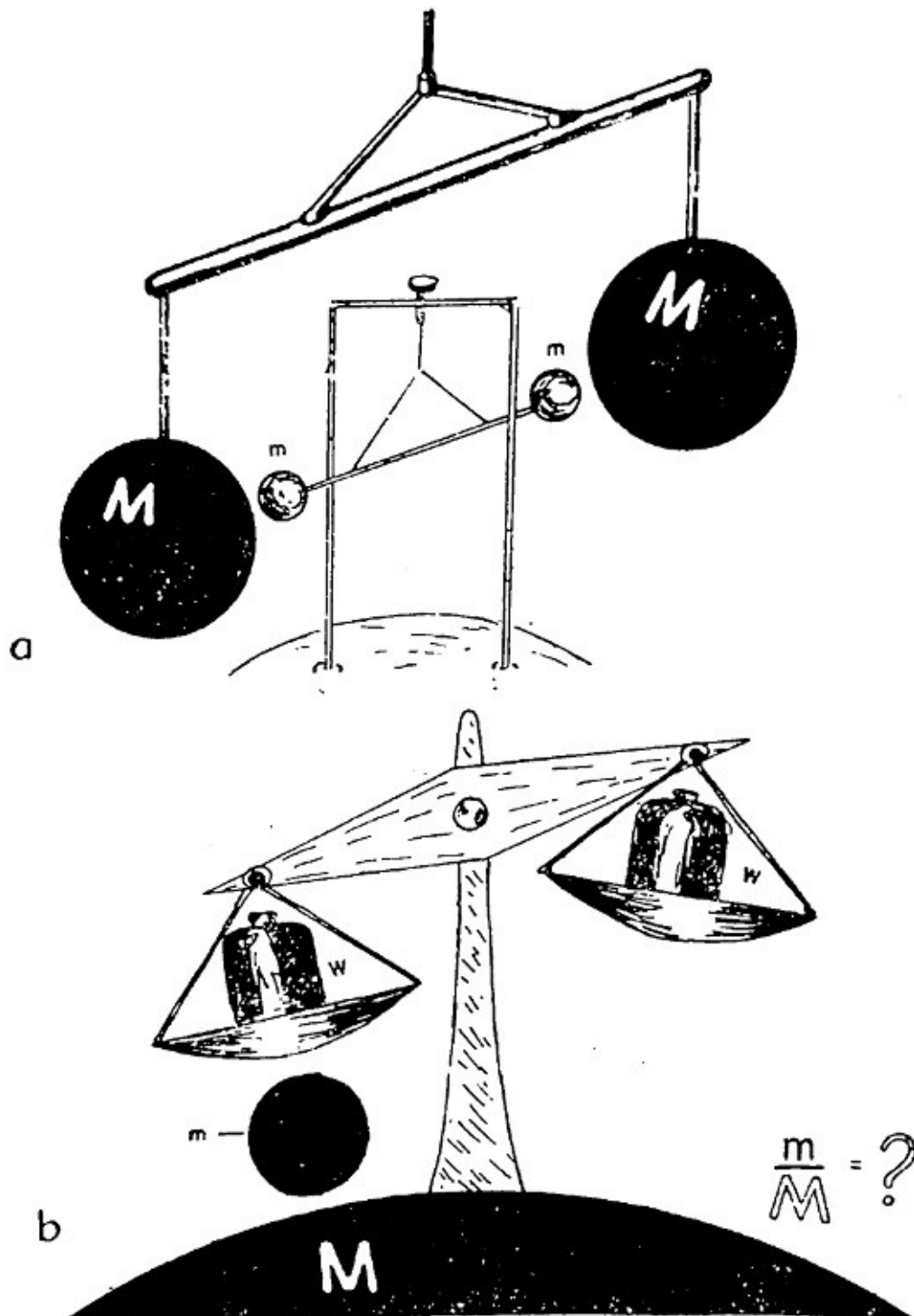
Figura 5.4. El aparato de Cavendish para medir la atracción gravitatoria era semejante al aparato de Coulomb para medir las fuerzas eléctricas. Cambiando la posición de dos grandes masas M suspendidas del techo (a), se observa el desplazamiento de dos masas más pequeñas m suspendidas de un hilo muy fino. b) Muestra la modificación del método de Cavendish; dos pesos W , previamente en equilibrio bajo
