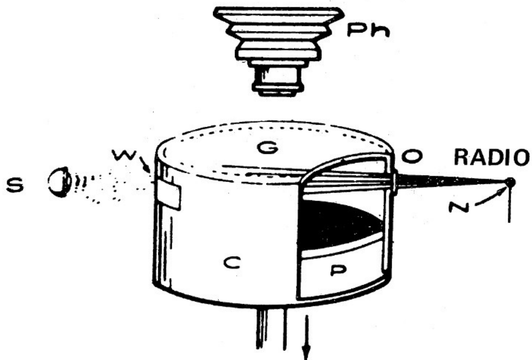
Figura 8.8. Esquema de la cámara de niebla de C. T. R. Wilson
