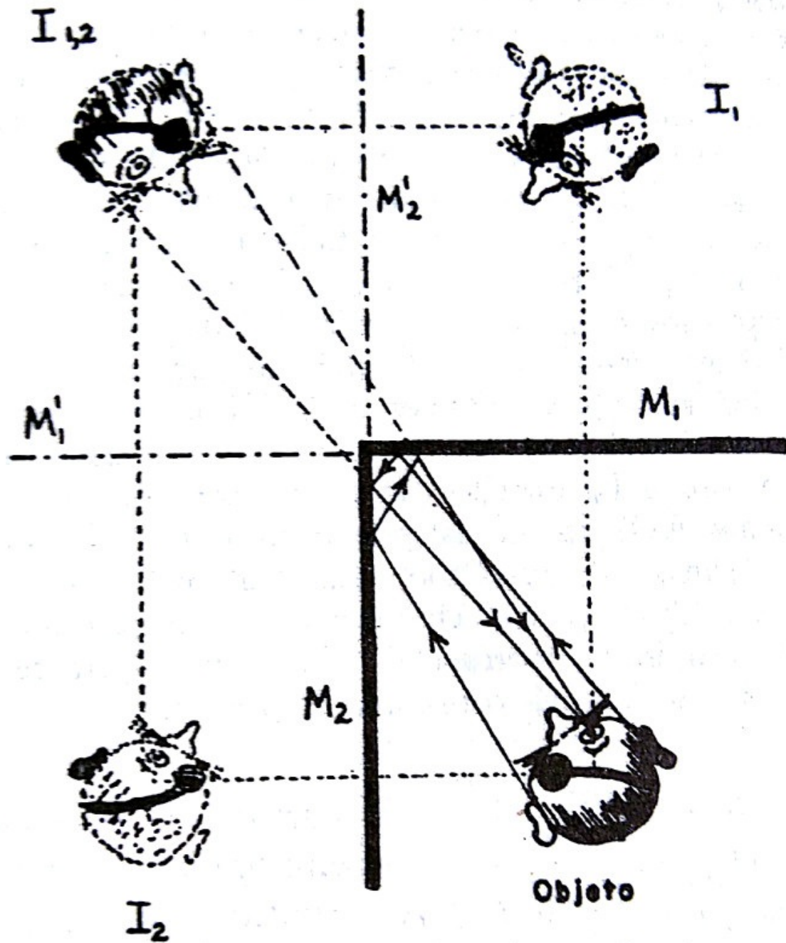
Figura 1.9. Mirando en un espejo compuesto formado por dos espejos planos, M_1 y M_2 , colocados borde contra borde en ángulo recto, se ve una imagen doblemente reflejada: primero en el espejo M_1 y después en la continuación imaginaria M'_2 del espejo M_2 , o primero en el espejo M_2 y después en la continuación imaginaria M'_1 del espejo M_1 . A causa de la doble reflexión, el lado derecho sigue siendo el derecho y el lado izquierdo el izquierdo. Los rayos de luz se representan por líneas llenas.
