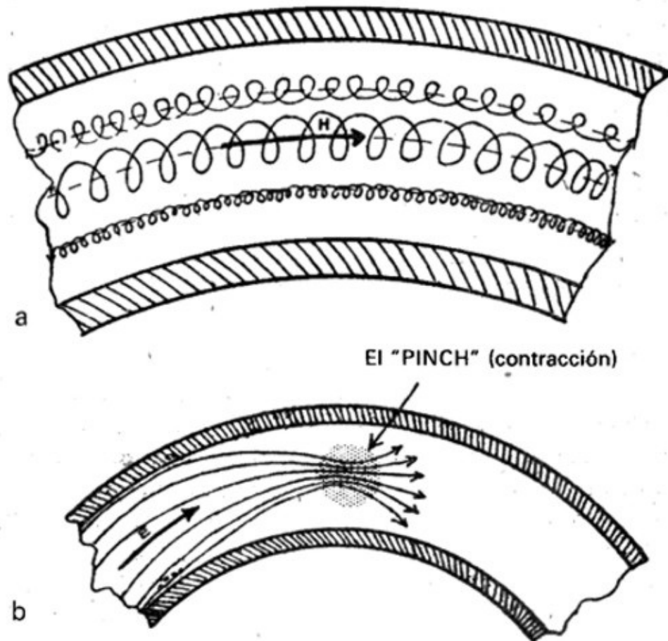
Figura 8.18. Los dos métodos principales que se están desarrollando actualmente para controlar las reacciones termonucleares. «Stellarator» en Princeton y «Perhapsotron» en Los Álamos.
