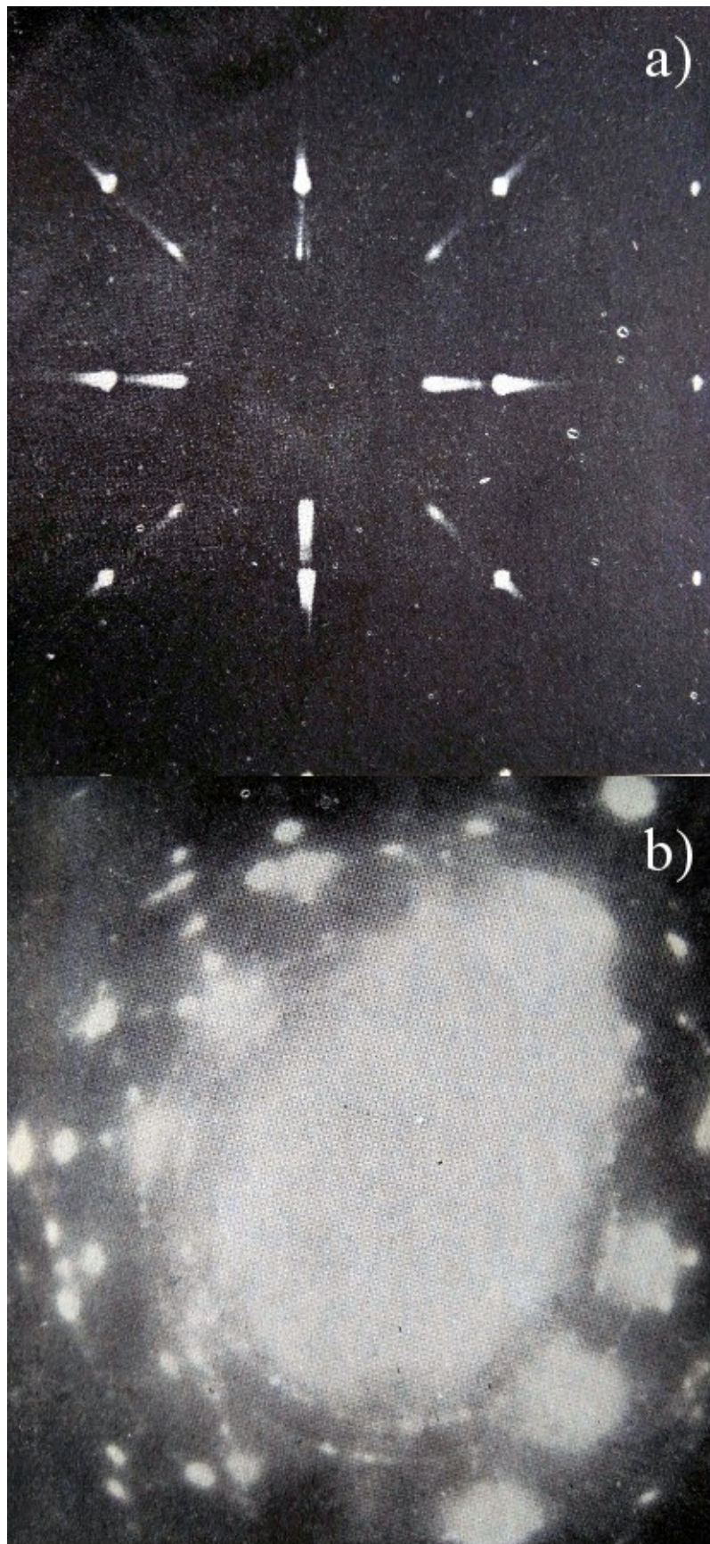
Lámina IV. a) Difracción de rayos X por una aleación de hierro y níquel. b) Difracción de electrones de 100 kW en la misma aleación que en a).
