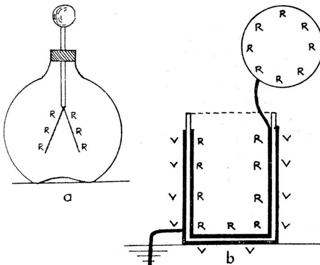
Figura 5.1. a) Electroscopio de panes de oro. b) Botella de Leyden.
