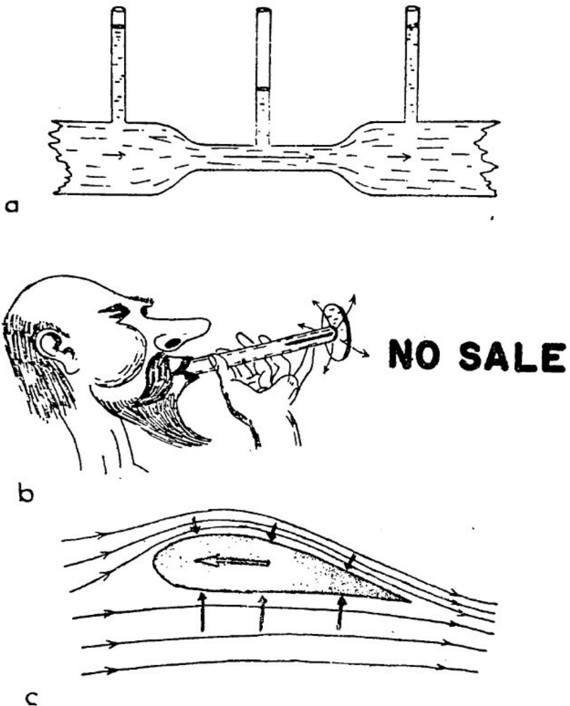
Figura 3.8. Principio de Bernoulli: a) Una demostración sencilla. b) El truco del tubo. c) Cómo actúan las alas de un avión.
