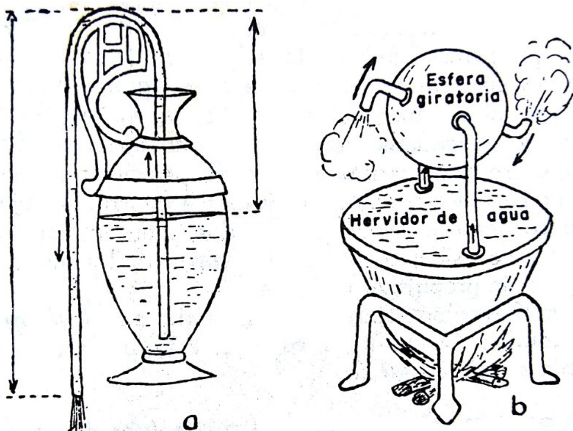
Figura 1.8. Dos aparatos inventados por Herón: a) el sifón permite que el agua de una vasija se derrame por sí sola a través de un tubo encorvado. La razón de que el agua salga por el tubo es que el peso del agua en la parte larga de la izquierda del tubo es mayor que el peso del agua en la parte derecha, que se extiende tan sólo desde la superficie del agua en la vasija hasta lo alto del tubo; b) el aparato de reacción a chorro, en el cual la rotación de la esfera se produce por los dos chorros de vapor que salen por las toberas.
