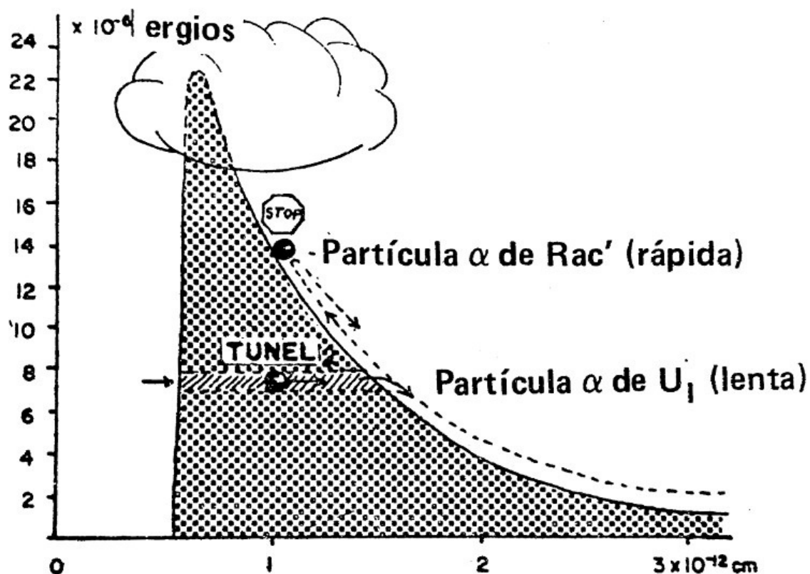
Figura 8.3. La barrera de potencial en torno al núcleo de uranio tal como resulta de los experimentos de dispersión de Rutherford.
