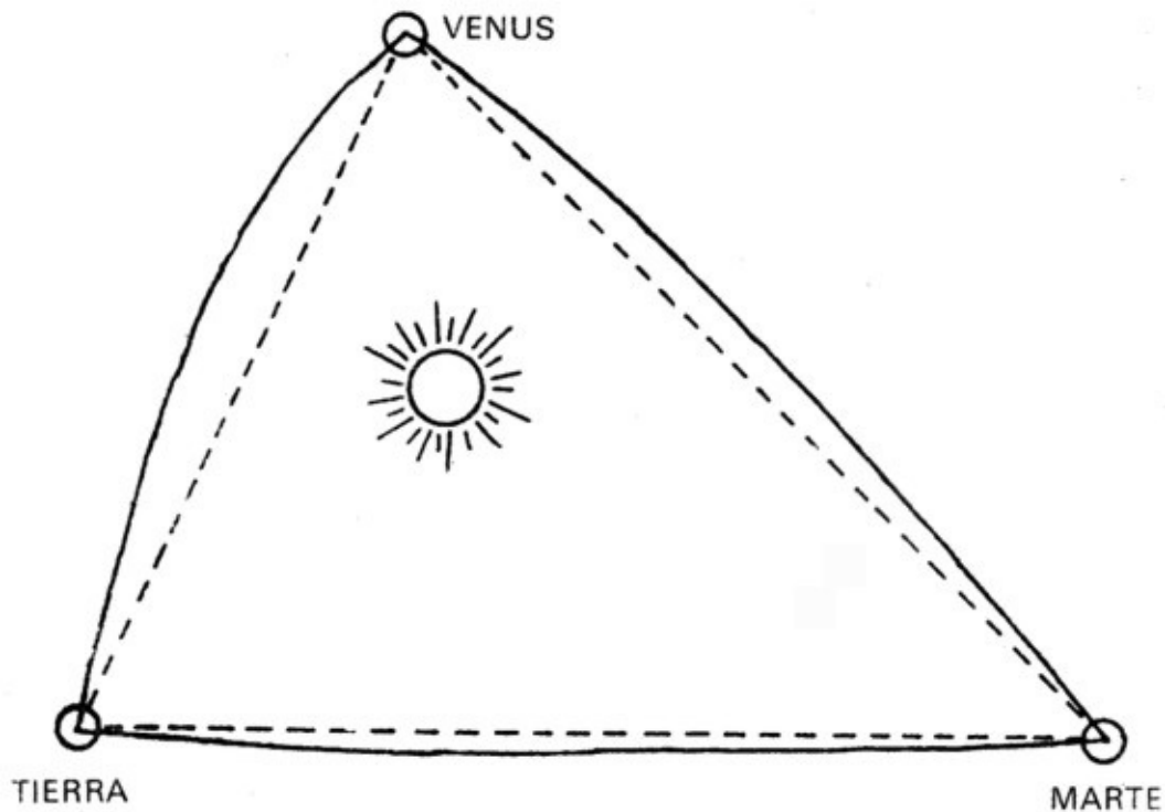
Figura 6.14. Triangulación del espacio en torno al Sol.
