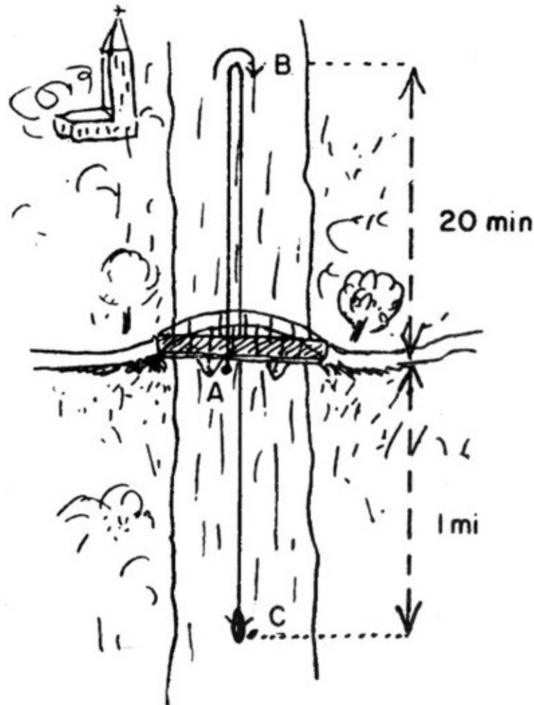
Figura 6.5. Problema de la recuperación de una botella arrojada al agua.
