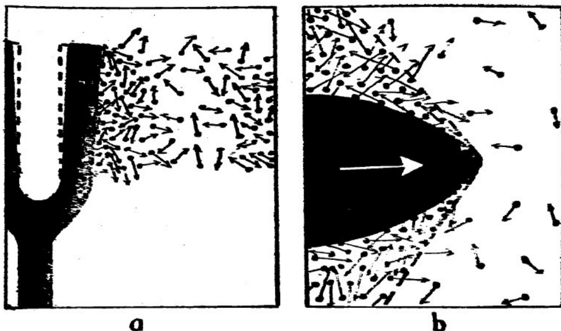
Figura 4.21. Formación de una onda sonora en el caso en que el elemento que empuja se mueve más lentamente que las moléculas a), y la formación de ondas de choque cuando se mueve más rápidamente b).
