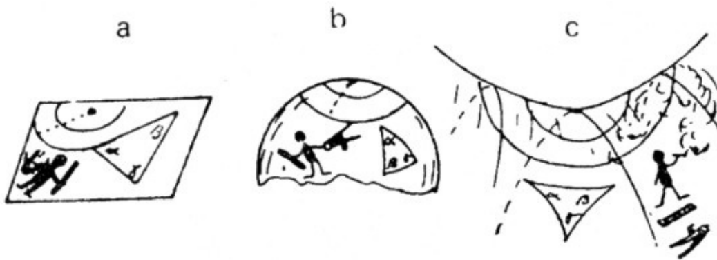
Figura 6.13. Tres diferentes tipos de superficies (dos dimensiones) curvas. a) Superficie plana: curvatura cero. b) Superficie esférica: curvatura positiva. c) Superficie de silla de montar: curvatura negativa. La diferencia entre los tres casos puede ser descubierta por seres inteligentes bidimensionales si estudian la geometría de los círculos o triángulos.
