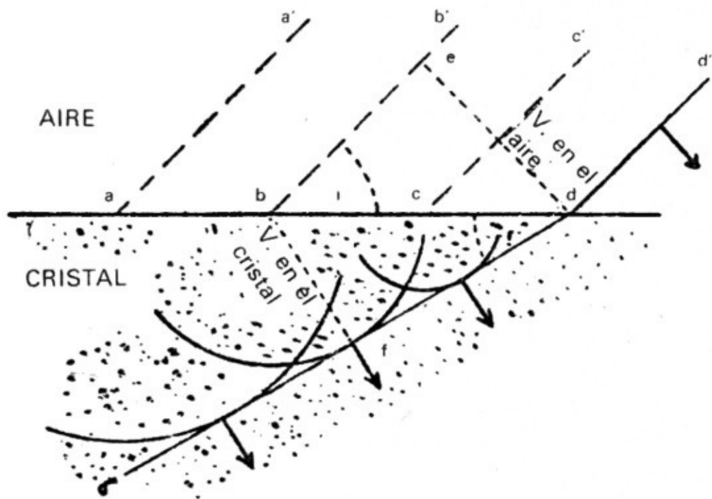
Figura 3.16. Explicación de Huygens de la refracción de la luz.
