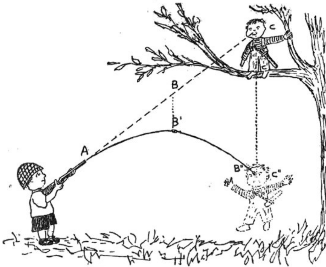
Figura 2.7. Como todos los cuerpos caen con la misma aceleración, si un niño que juega con otro a la guerra de la selva dispara un proyectil directamente al «enemigo», situado en la rama de un árbol, la bala dará exactamente en la nariz de este último, si se deja caer en el momento del disparo.
