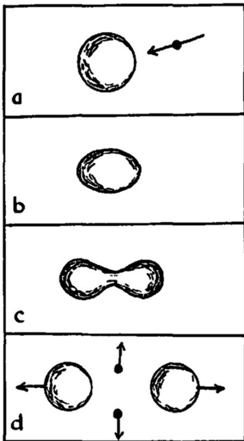
Figura 8.14. Fisión de un núcleo pesado a consecuencia del impacto de un neutrón.
