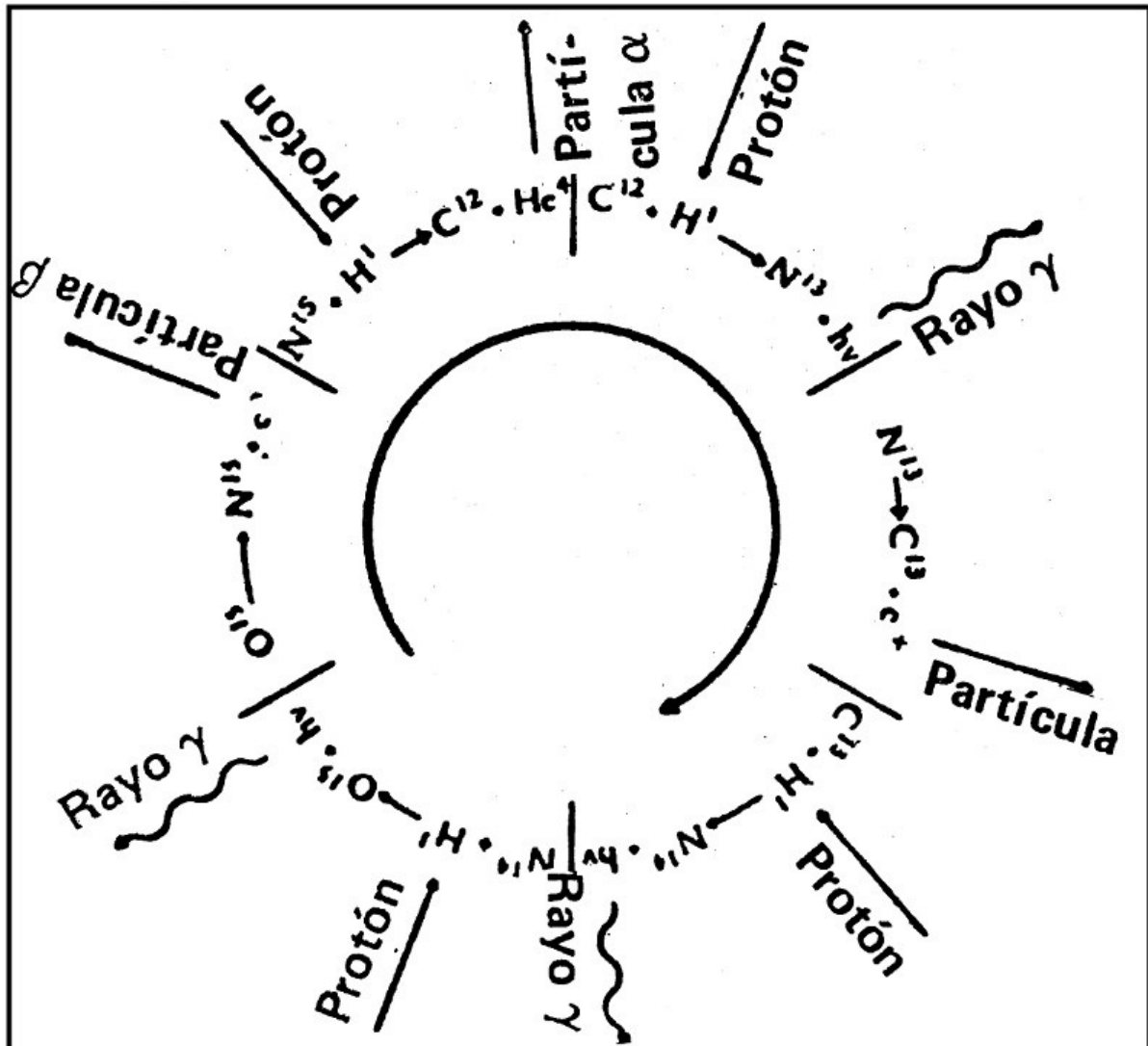
Figura 8.15. Ciclo de carbono responsable de la energía termonuclear en las estrellas.
