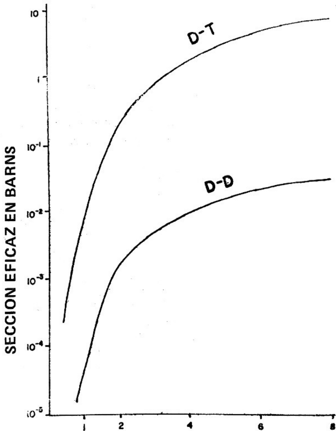
Figura 8.16. Secciones eficaces para las reacciones D-D y D-T como función de su energía térmica expresada en términos de temperatura absoluta.
