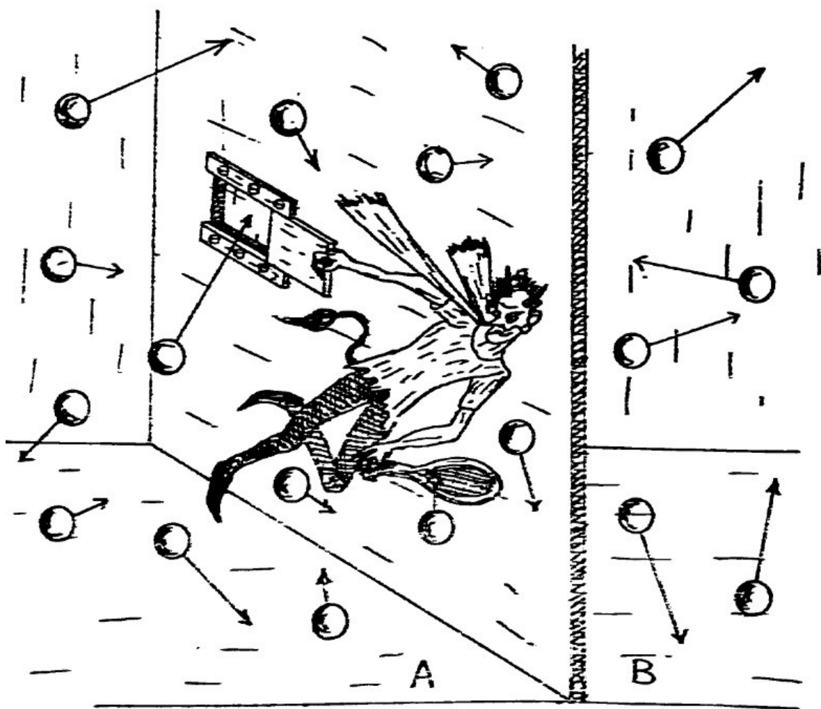
Figura 4.10. El demonio de Maxwell, que se supone puede separar las moléculas rápidas y lentas.
