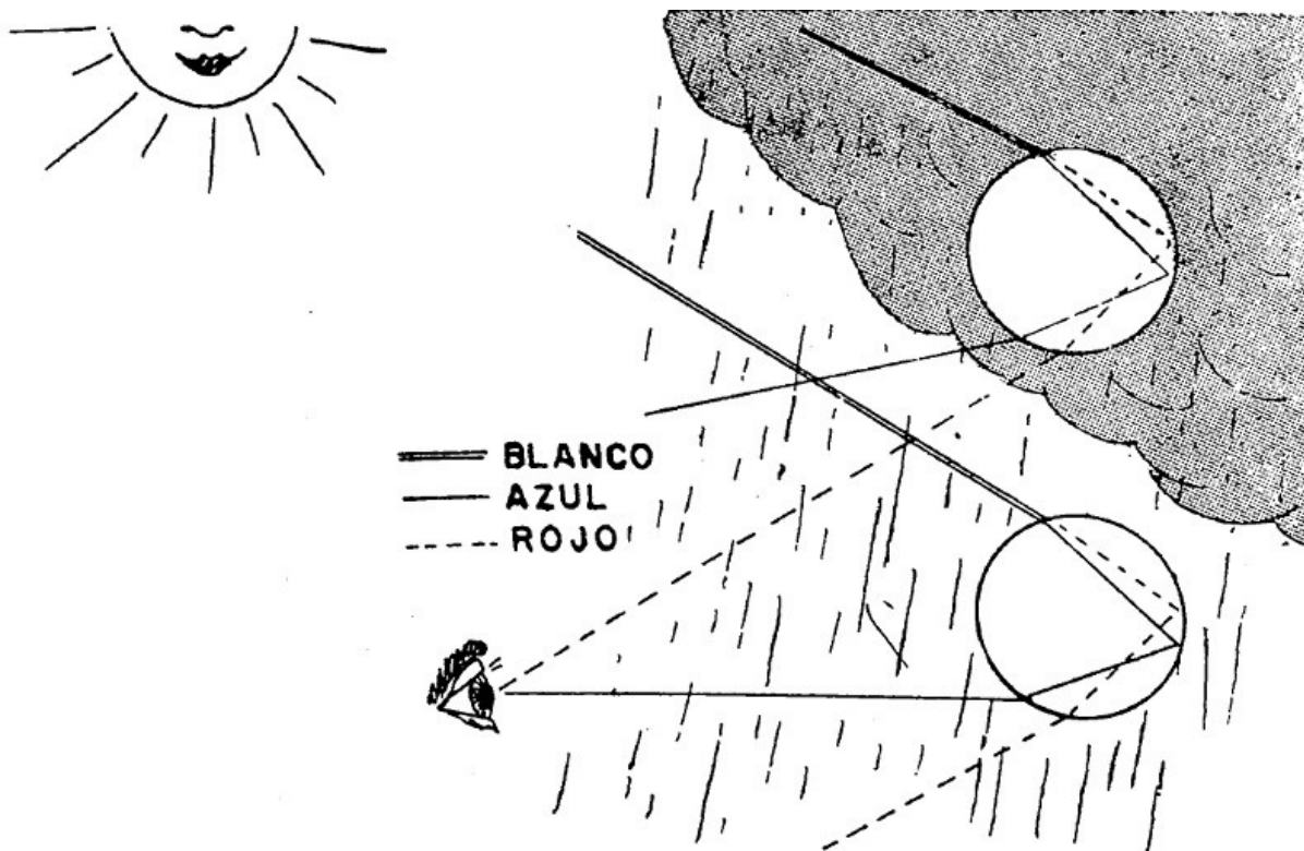
Figura 3.11. Explicación de Newton de los colores del arco iris.
