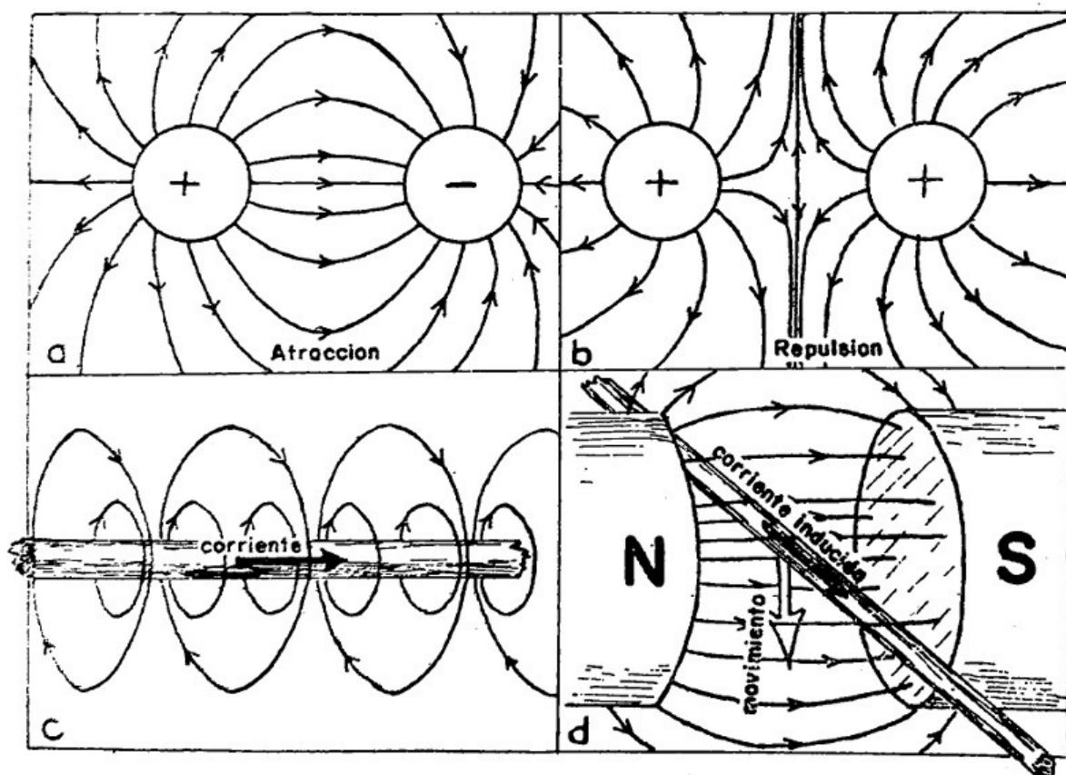
Figura 5.15. Líneas de fuerza de Faraday correspondientes a diferentes tipos de interacciones electromagnéticas: a) Líneas de fuerza eléctrica entre dos cargas eléctricas contrarias. b) Líneas de
