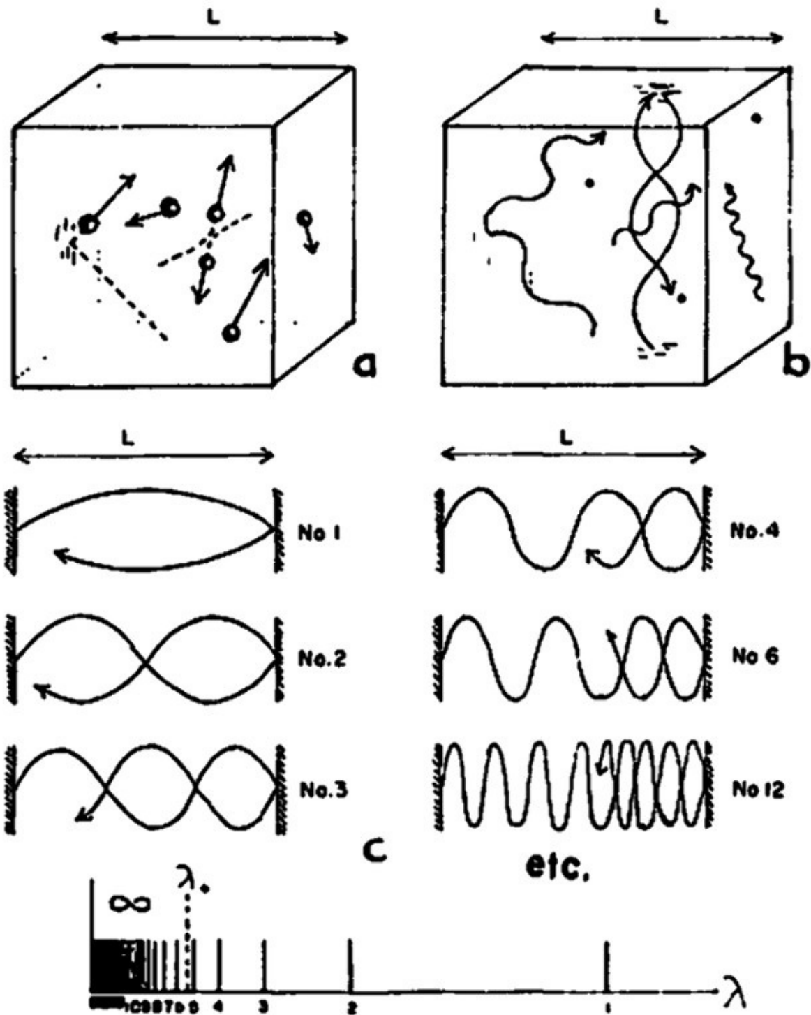
Figura 7.8. Comparación entre el movimiento al azar de las moléculas de gas en un recinto cerrado (a) y el movimiento al azar de las ondas en el cubo de Jeans (b). Los puntos negros en (b) representan diminutas partículas de polvo de carbón que sirven como cambiadores de energía entre las ondas. (c) Representa varios modos de vibraciones en el cubo de Jeans (en el caso de una dimensión para mayor simplificación) mientras (d) representa el espectro correspondiente.
