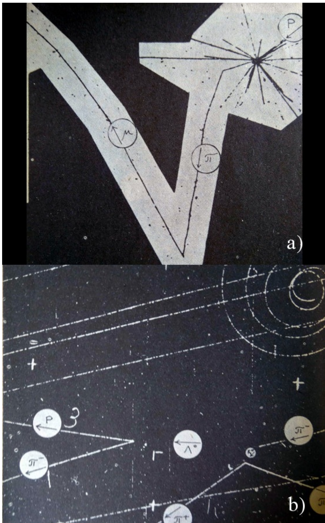
Lámina VIII. a) Formación de un pion y su posterior desintegración en un muón y un electrón. Foto con emulsión gruesa. b) Una serie de sucesos nucleares en una cámara de burbujas.
