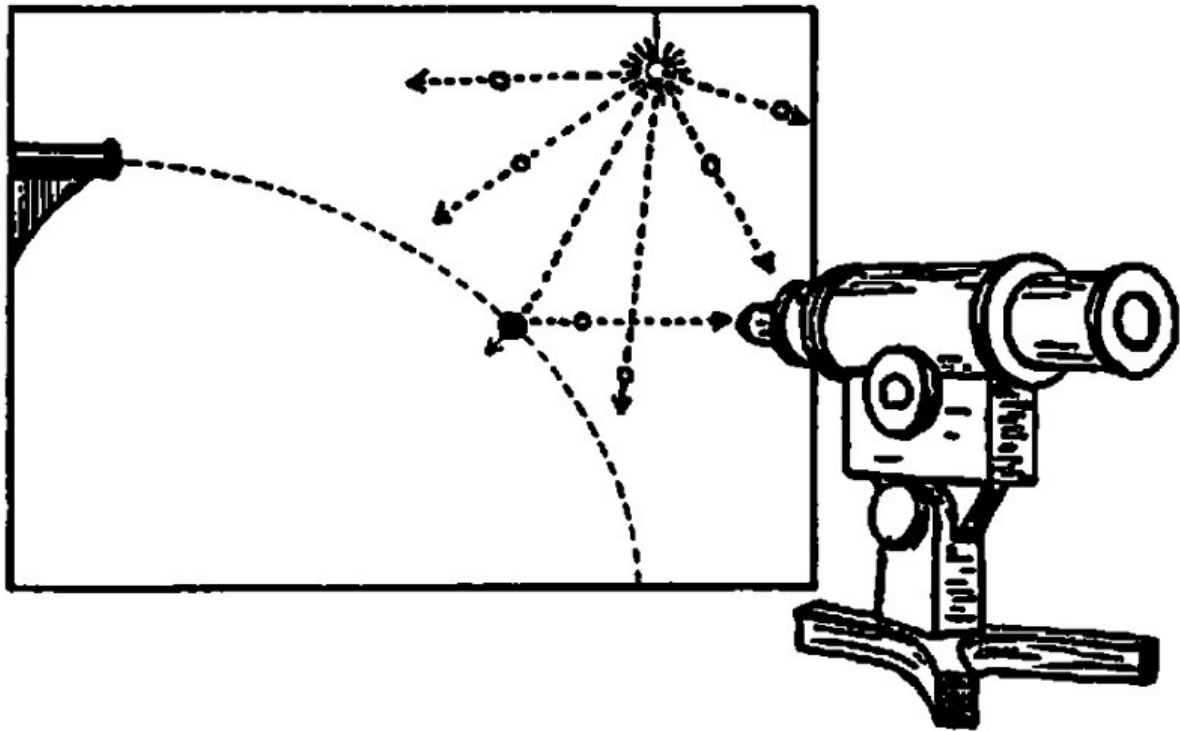
Figura 7.20. Experimento ideado por Heisenberg para observar la trayectoria de una partícula.
