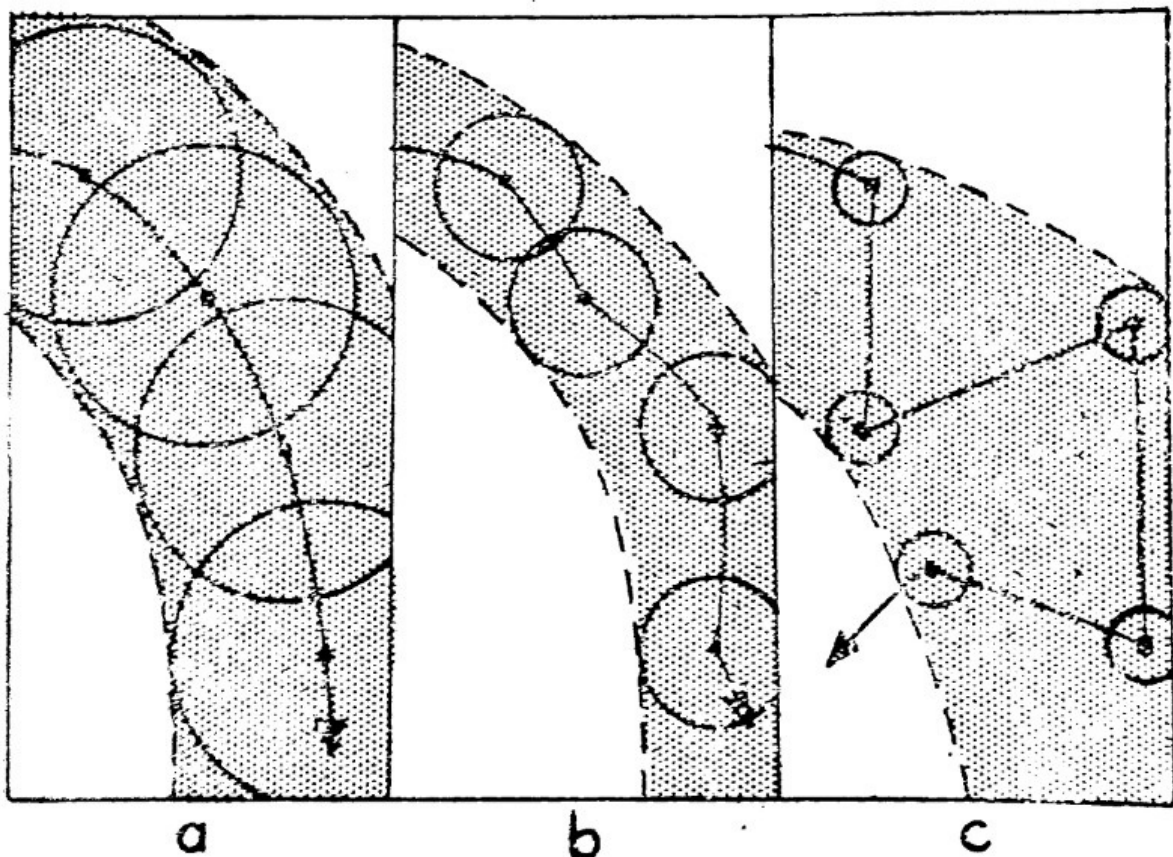
Figura 7.21. La trayectoria de una partícula en el experimento imaginario de Heisenberg. a) La longitud de onda de la luz es demasiado grande y la medición de cada posición es muy inexacta. b) Condiciones
