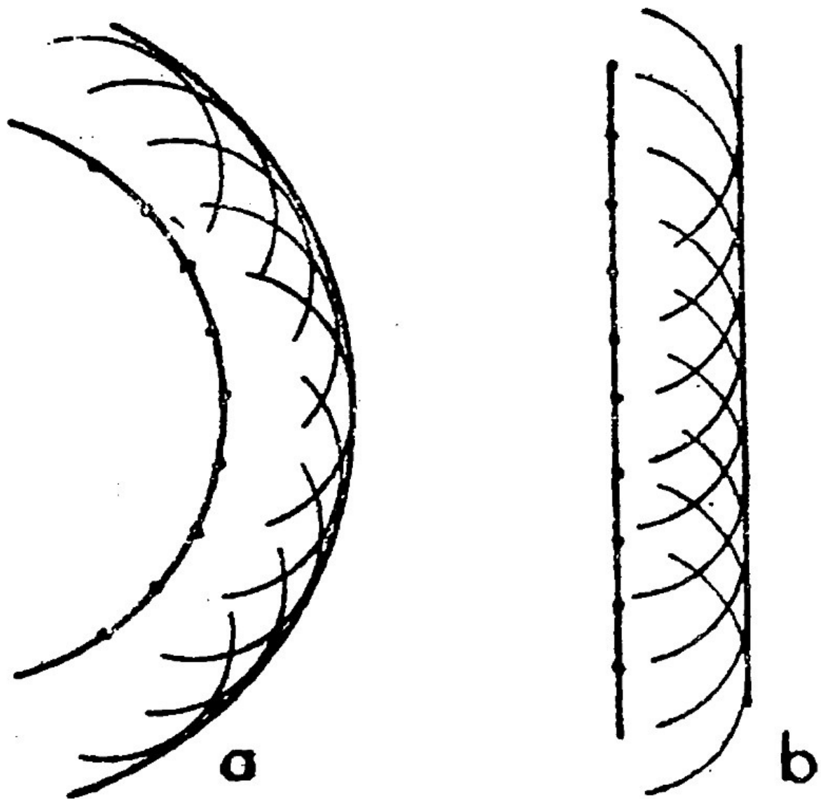
Figura 3.15. Principio de Huygens de la propagación de las ondas.
