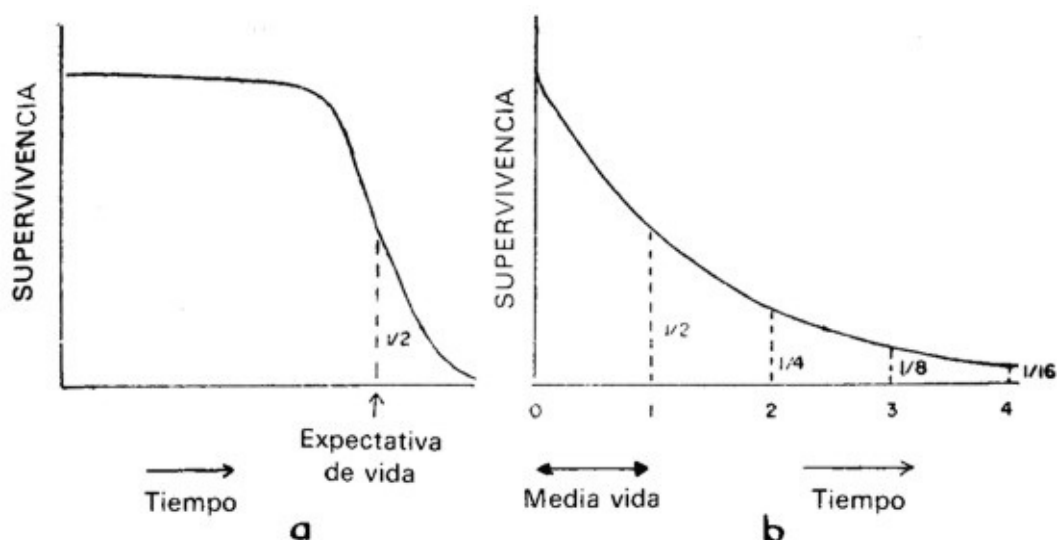
Figura 8.2. Curvas de supervivencia de animales (a) y núcleos (b).
