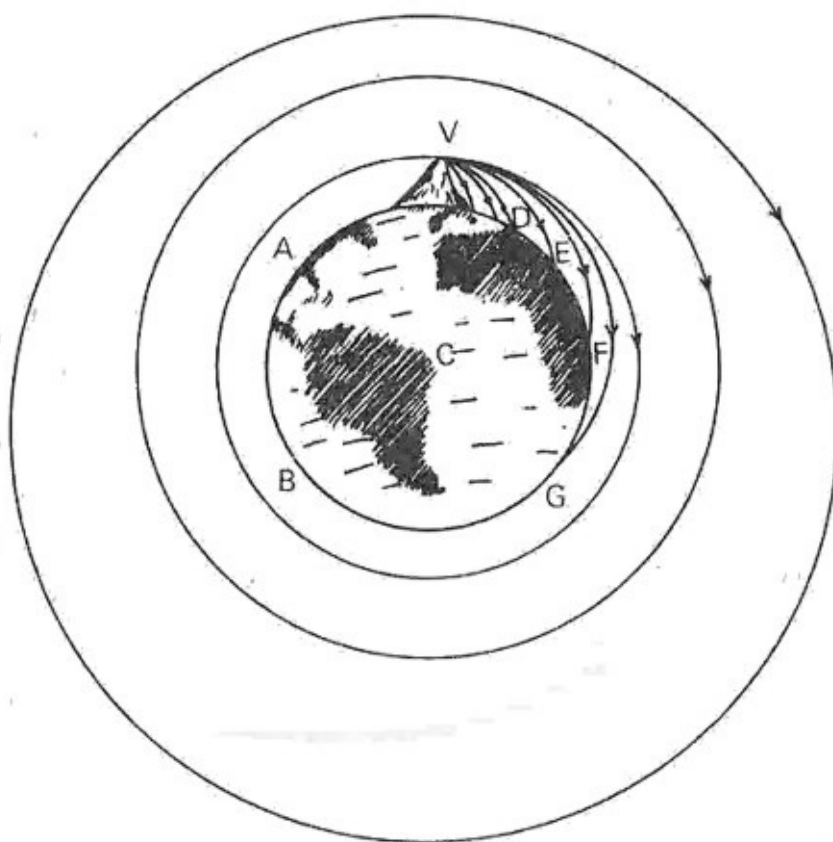
Figura 3.2. La trayectoria del satélite de la Tierra como caso límite de las trayectorias de proyectiles que caen cada vez a más distancia de la base de la montaña de la cual fueron arrojados. (Adaptación del dibujo original inserto en los Principia de Newton.)
