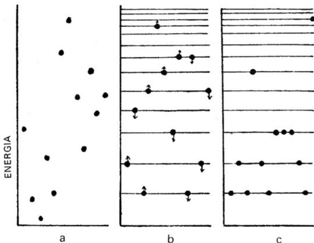
Figura 7.24. Tres clases de tratamiento estadístico de la energía de doce partículas de gas.
