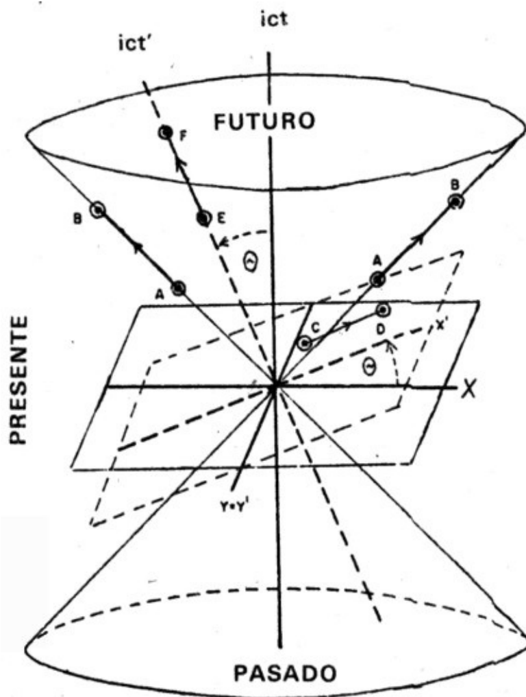
Figura 6.11. El continuo espacio-tiempo, con dos coordenadas de espacio ( x e y ) y la coordenada de tiempo ( ict ). Las superficies cónicas que representan la propagación de la luz ( x^2 + y^2 - c^2t^2 = 0 ) dividen el continuo en «presente», «pasado» y «futuro».
