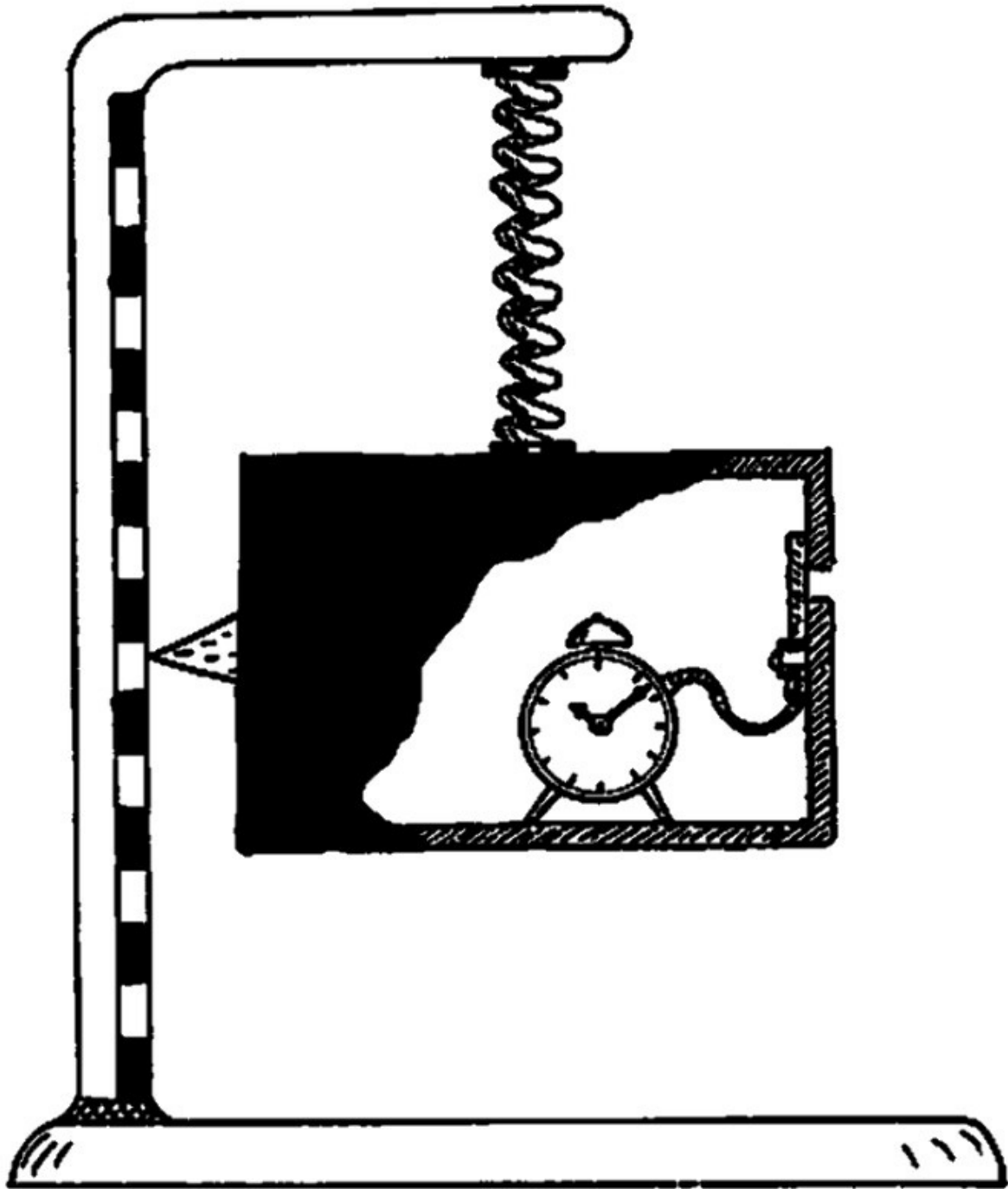
Figura 7.22. Balanza de Einstein-Bohr para medir el peso de la luz.
