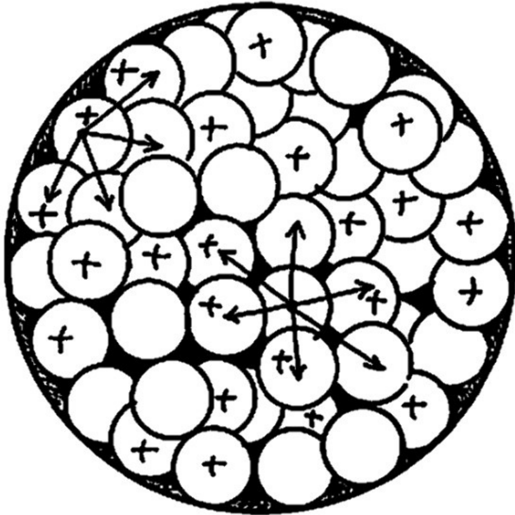
Figura 8.11. Núcleo atómico compuesto de protones y neutrones. Los que están en el interior no experimentan ninguna fuerza, mientras los de la superficie son impelidos hacia el centro.
