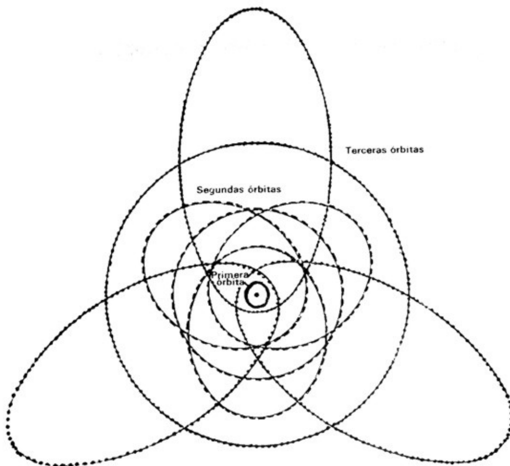
Figura 7.14. Órbitas cuánticas circulares y elípticas en el átomo de hidrógeno. La primera órbita circular (línea llena) corresponde a la menor energía del electrón. Las siguientes cuatro órbitas, una circular y tres elípticas (líneas de trazos) corresponden a la misma energía, mayor que en la primera órbita. Las siguientes nueve órbitas (líneas de puntos), de las cuales sólo cuatro aparecen en la figura, corresponden a una energía aún mayor (la misma para las nueve).
