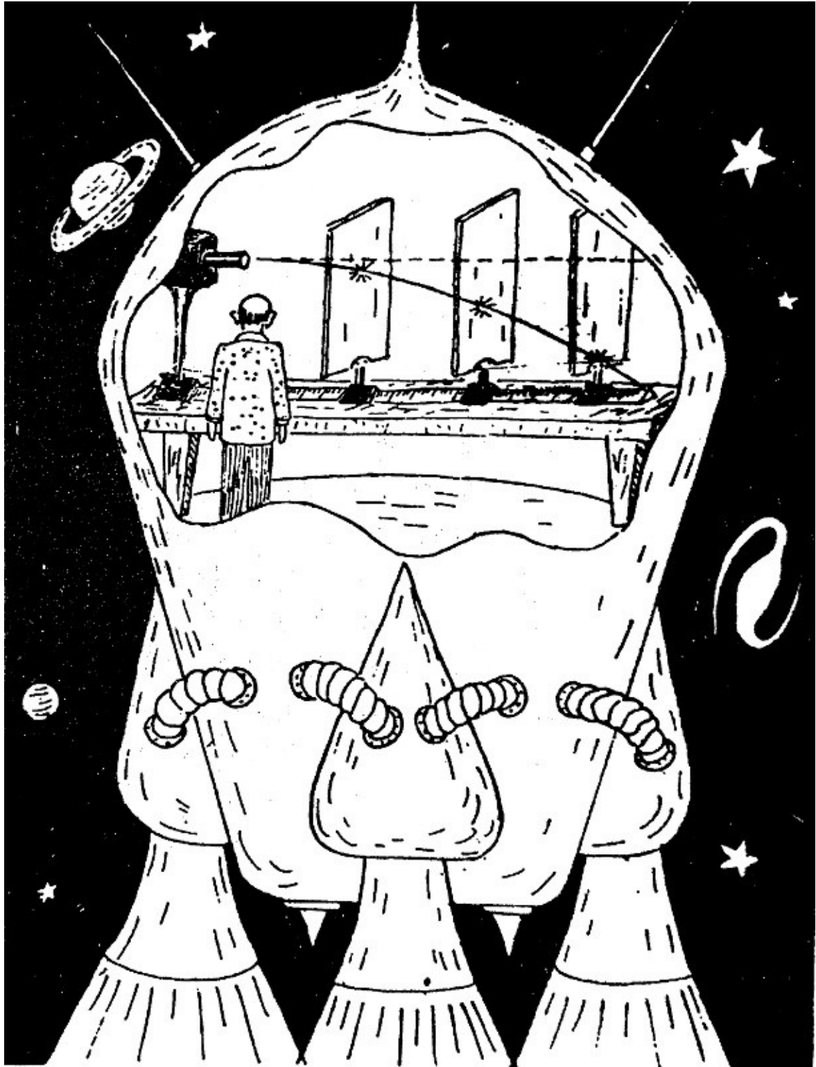
Figura 6.12. Experimento óptico en un cohete acelerado que indica que los rayos de luz pueden ser curvados por el campo gravitatorio.
