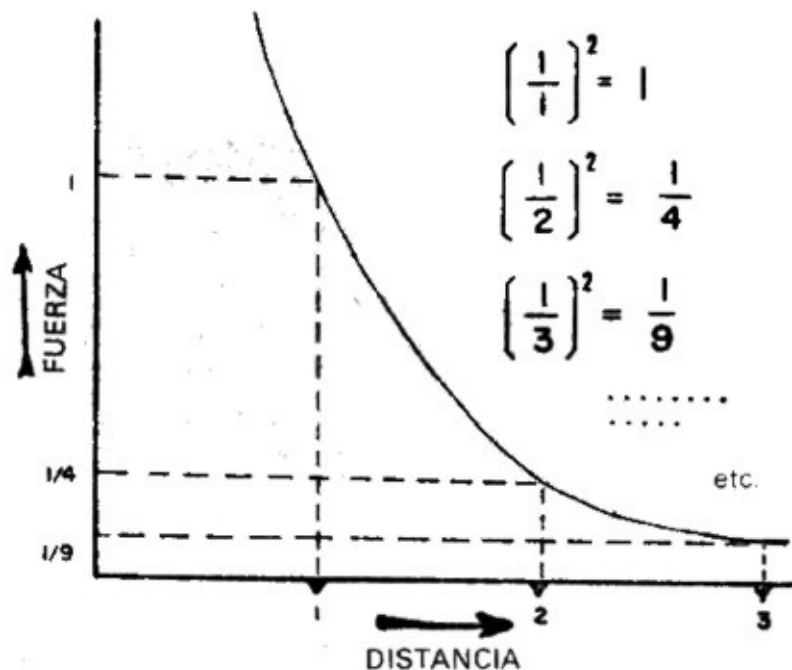
Figura 5.3. Un gráfico de la ley de Coulomb.
