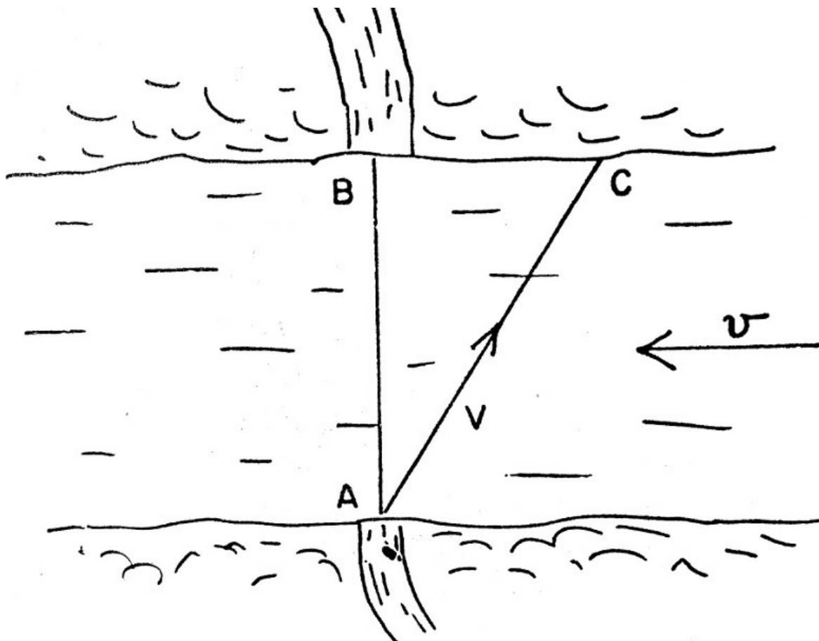
Figura 6.3. El problema de una lancha que cruza un río.
