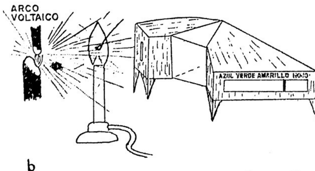
Figura 4.14. a) El sodio introducido en una llama caliente emite una característica línea amarilla. b) Cuando la luz blanca de un arco voltaico, que contiene todas las longitudes de onda, pasa a través de una llama que contiene sodio, aparece una línea oscura de absorción donde estaba antes la línea brillante de emisión.
