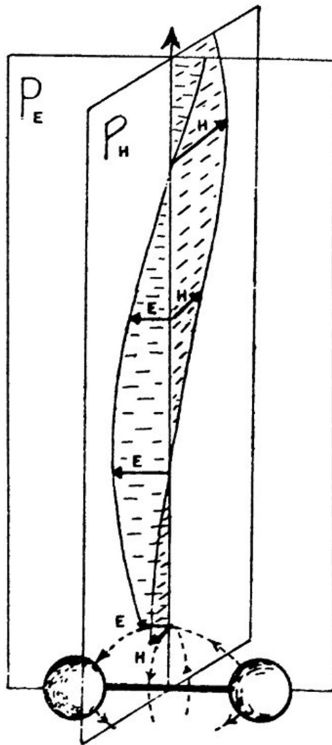
Figura 5.18. Formación de una onda electromagnética propagada como resultado de la oscilación de carga entre dos conductores.
