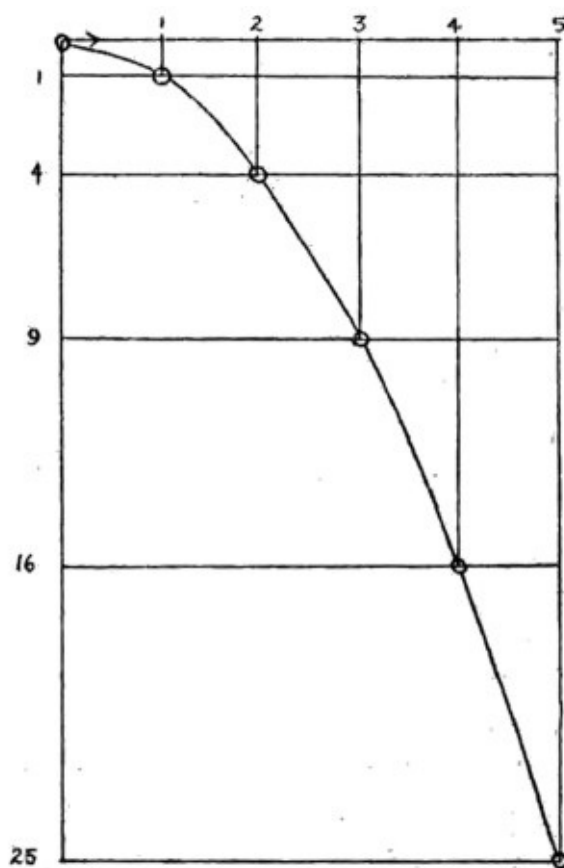
Figura 2.6. Composición de un movimiento uniforme en dirección horizontal y un movimiento acelerado en dirección vertical. La curva resultante es una parábola.
