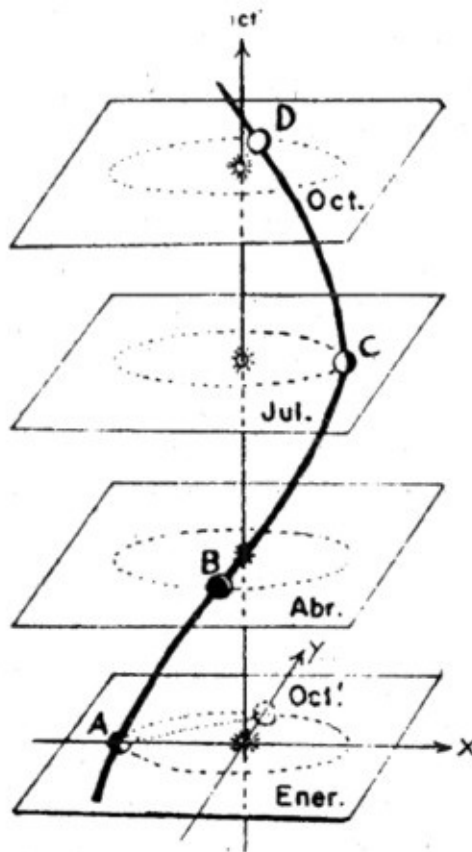
Figura 6.16. La línea cósmica de la Tierra en su movimiento alrededor del Sol, tratada en el sistema de coordenadas x, y, ict . La distancia dimensional espacio-tiempo entre las posiciones de la Tierra en enero y octubre es la distancia más corta. Pero la distancia entre la posición de enero y la proyección de la posición de octubre en el plano de enero ( Oct. ') no es evidentemente la más corta.
