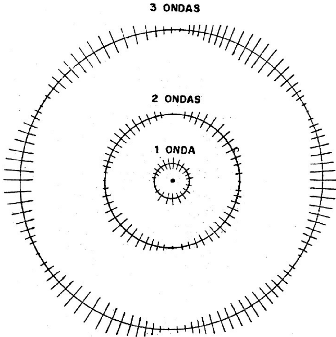
Figura 7.18. Ondas de De Broglie corriendo a lo largo de las órbitas de Bohr.
