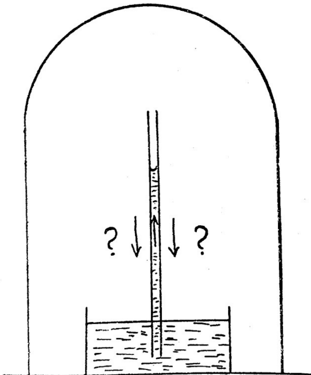
Figura 4.8. Un ejemplo de razonamiento termodinámico. Si la presión de vapor sobre el menisco cóncavo del tubo capilar fuera la misma que sobre la superficie del agua de la cubeta, el agua estaría en un estado de movimiento perpetuo en las direcciones indicadas por las flechas.
