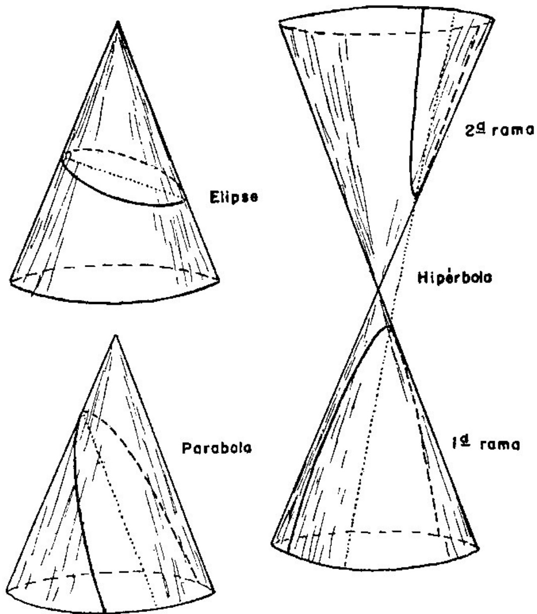
Figura 2.1. Secciones cónicas obtenidas cortando un cono por un plano en ángulos diferentes.
