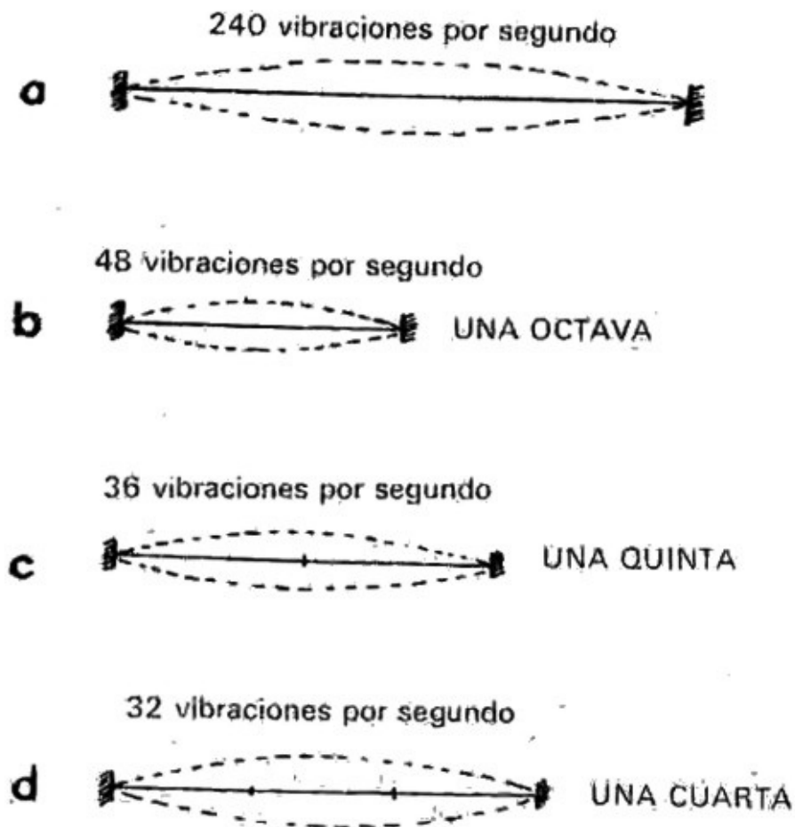
Figura 1.1. Ley pitagórica de las cuerdas.
