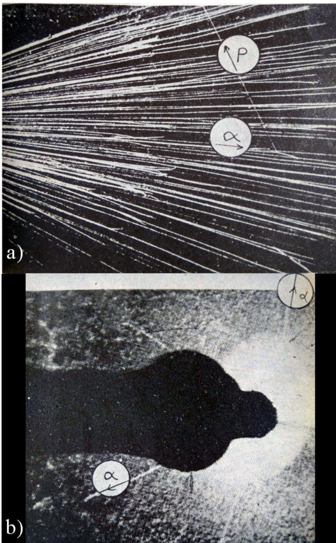
Lámina V. a) La primera fotografía de una transformación nuclear artificial en la cámara de niebla. b) La ruptura de un núcleo de boro en tres partículas alfa.
