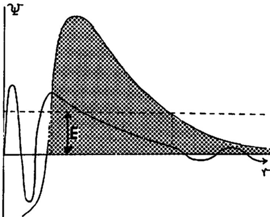
Figura 8.5. Penetración mecánico-ondulatoria de una partícula alfa a través de la barrera de potencial nuclear.
