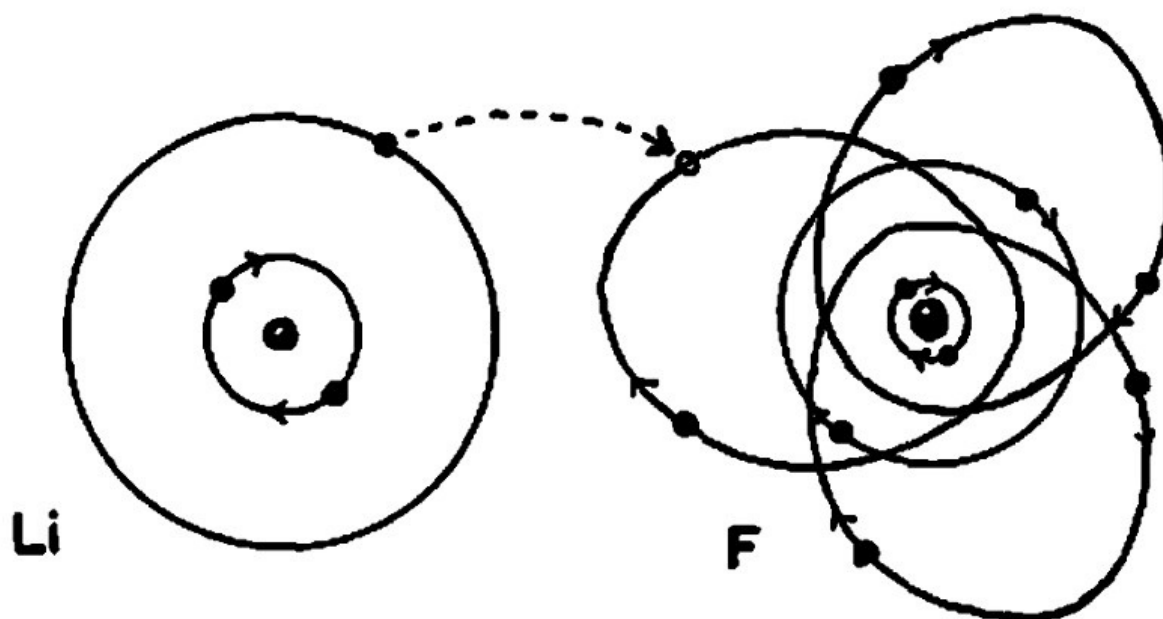
Figura 7.16. Enlace químico entre un átomo de litio (Li) y un átomo de flúor (F) en la molécula de fluoruro de litio (FLi). El electrón solitario de la capa exterior del litio salta a un lugar vacante de la
