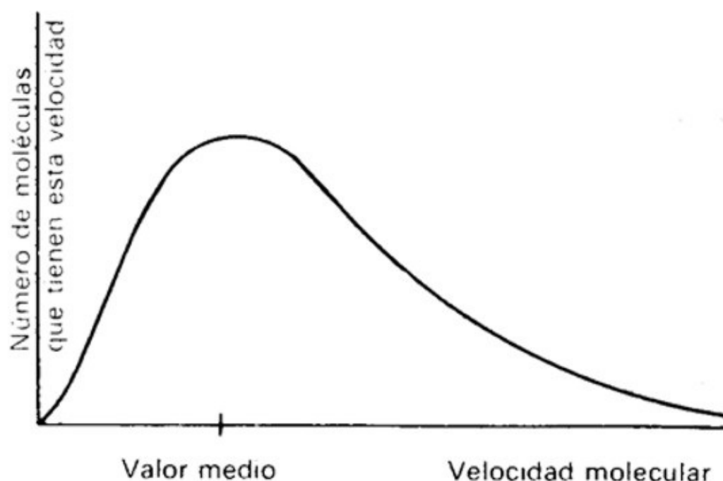
Figura 4.9. Curva de Maxwell de la distribución de velocidades.
