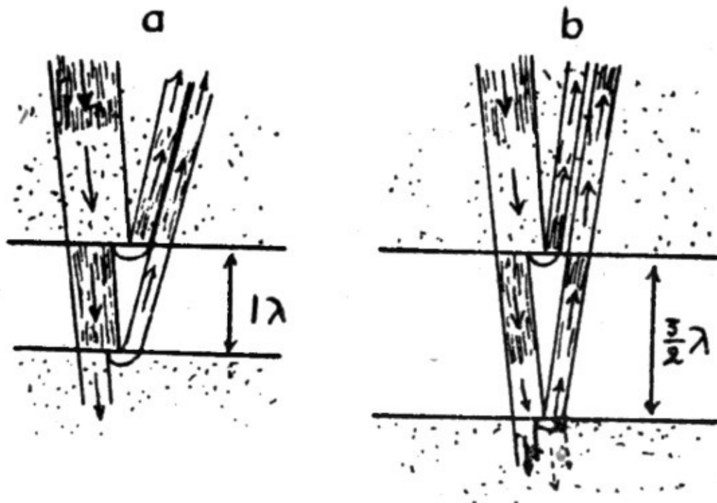
Figura 3.14. Explicación de Young de los anillos de Newton.
