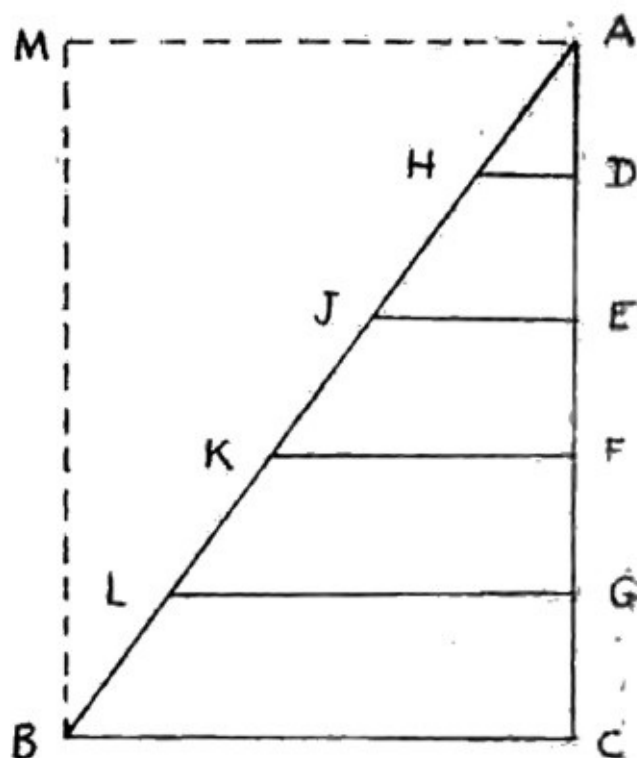
Figura 2.5. La prueba de Galileo de que en un movimiento (uniformemente) acelerado partiendo del reposo, la distancia recorrida por un móvil es la mitad de la distancia que el móvil habría recorrido si estuviera moviéndose todo el tiempo con la misma velocidad.
