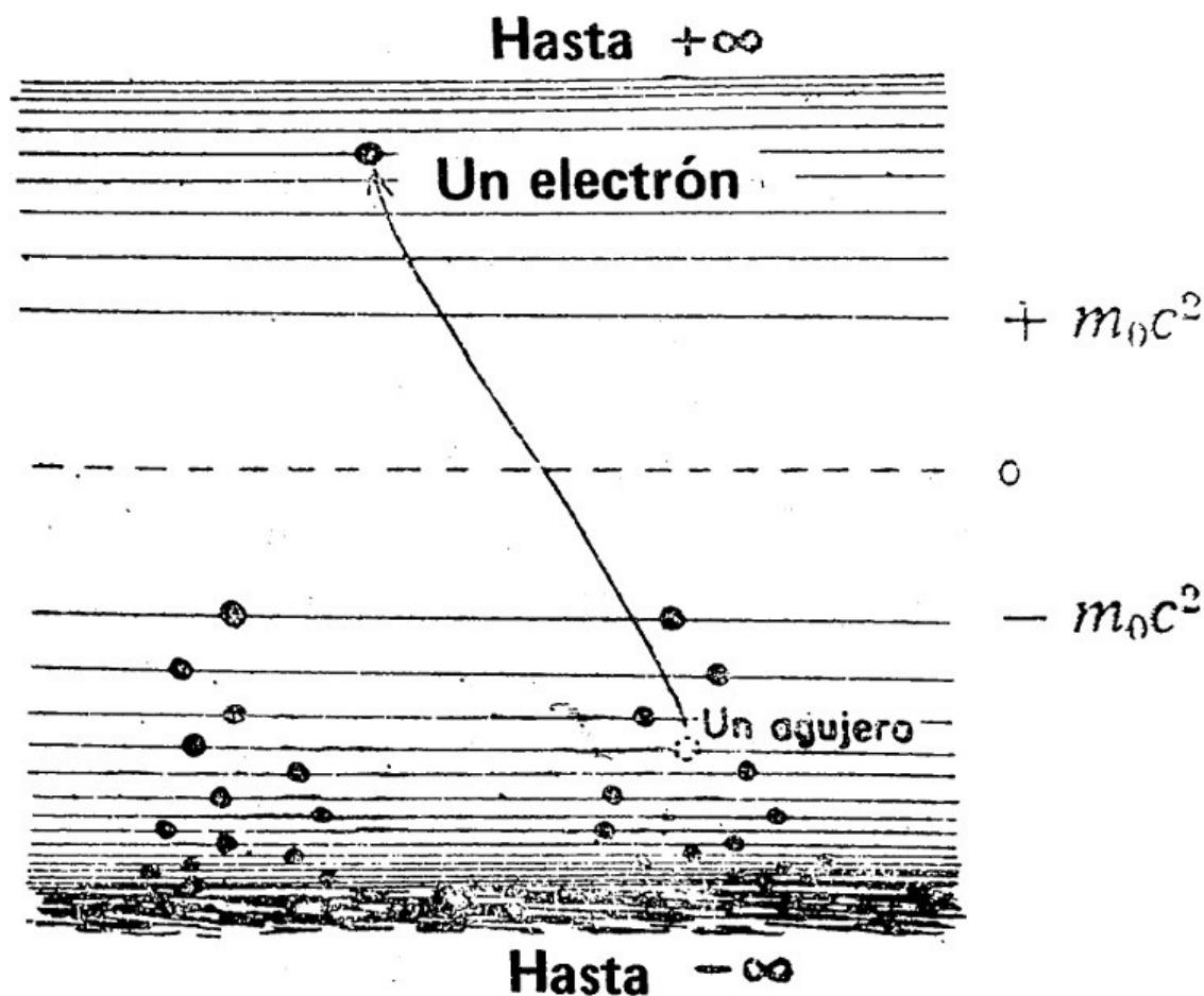
Figura 7.23. Océano de Dirac de «electrones pollinos» representando la formación de un par de electrones (uno positivo y otro negativo).
