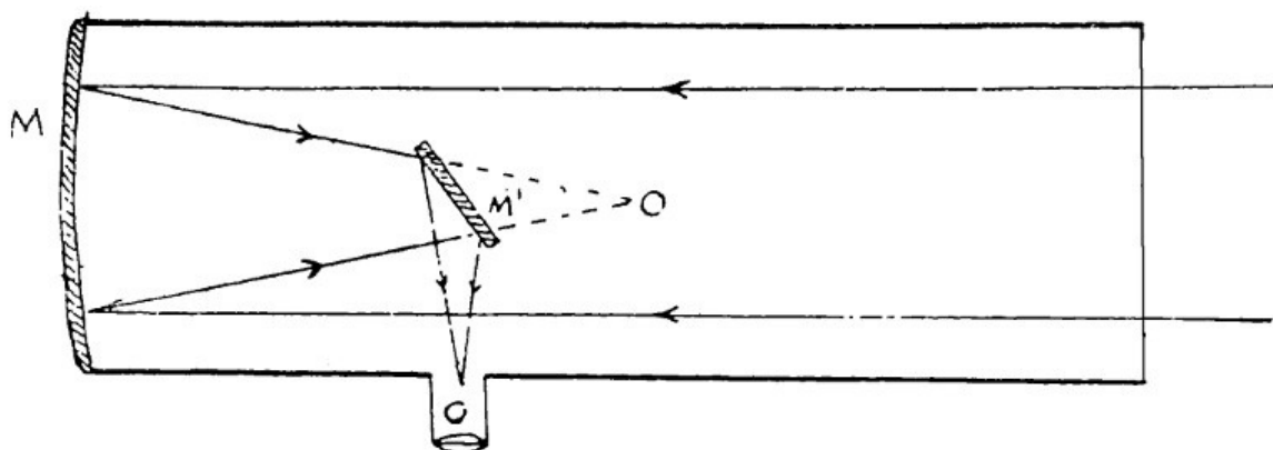
Figura 3.12. Telescopio de reflexión de Newton.
