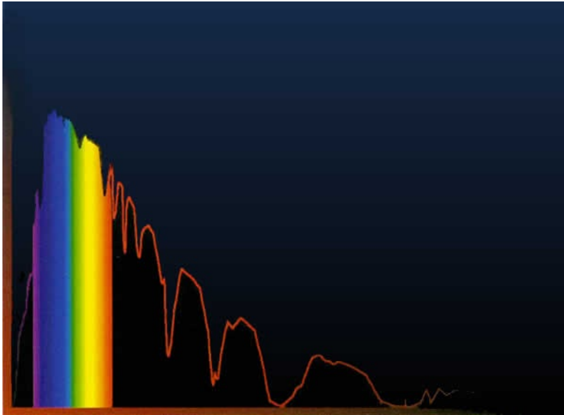
Espectro estelar
